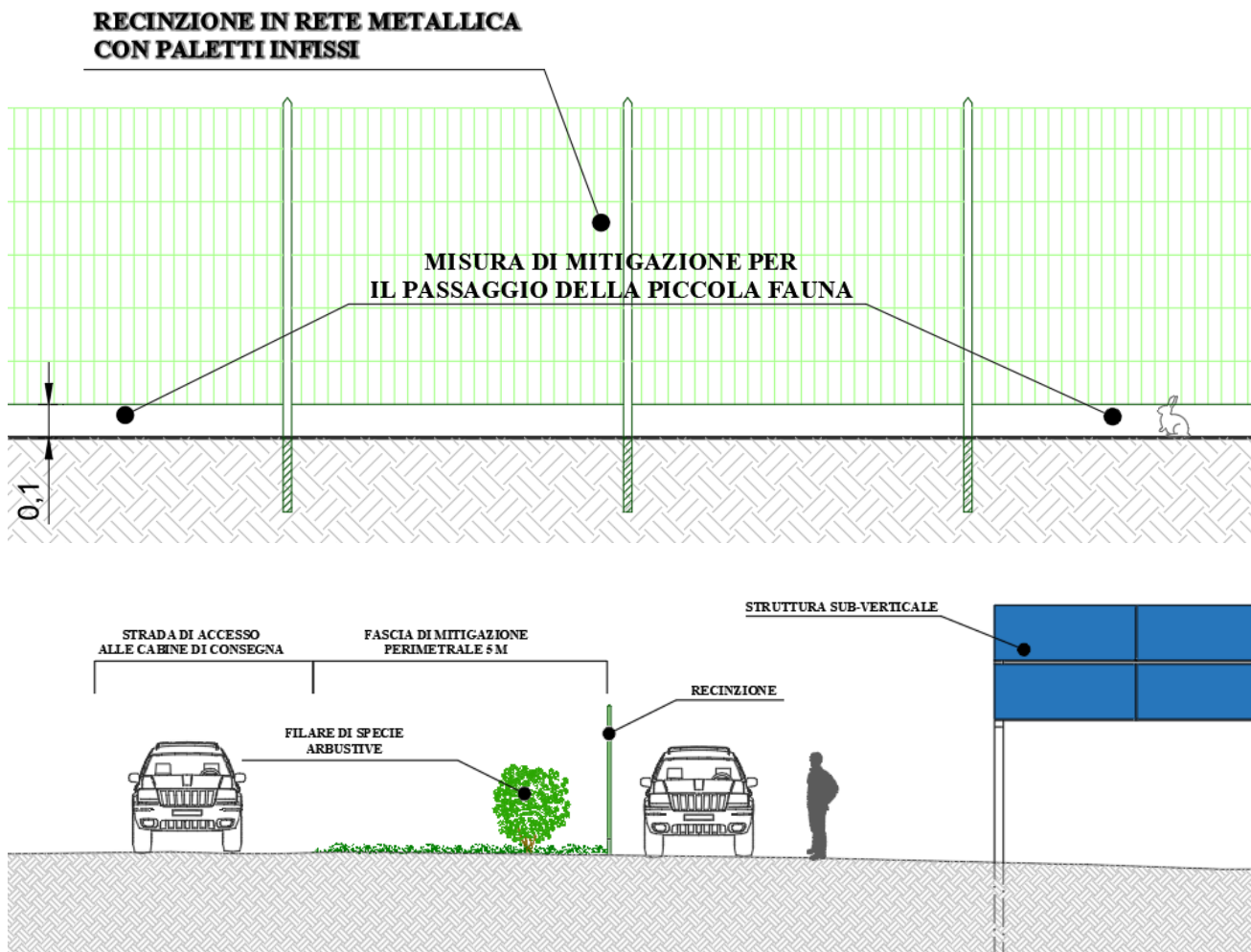
Figura 48 - Particolari della recinzione
