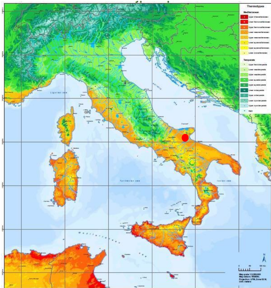
Figura 3 - Indice bioclimatico
