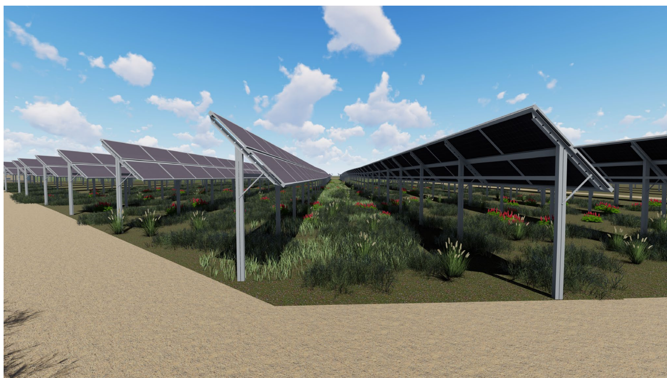
Figura 43 – Render area interna all'impianto – moduli fotovoltaici su strutture sub-verticali fisse
