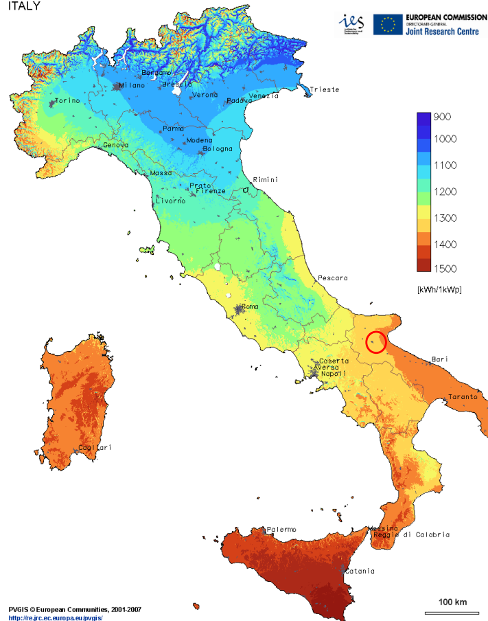
Figura 7 - Producibilità globale
