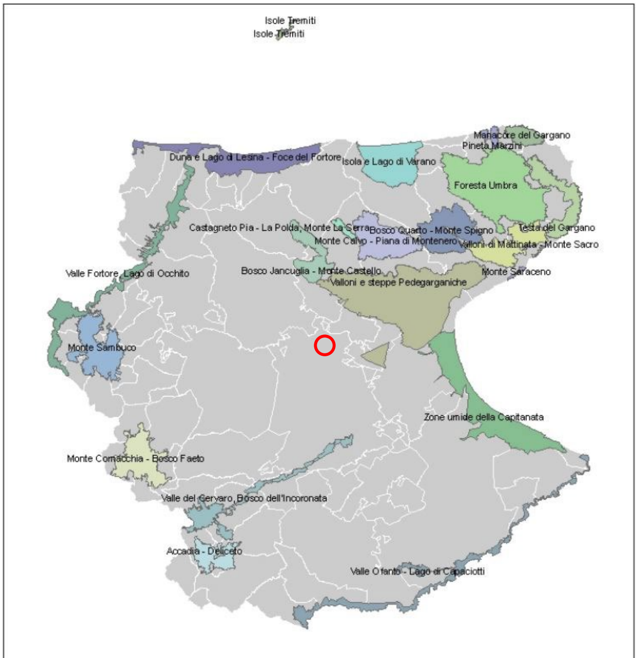
Figura 28 - SIC
