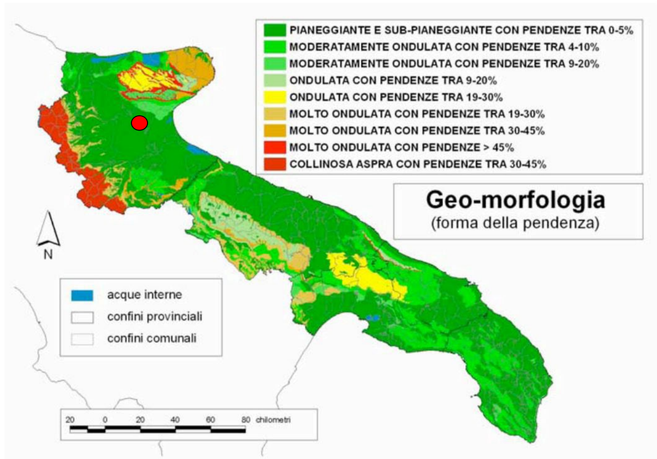
Figura 3 Carta geo-morfologia
