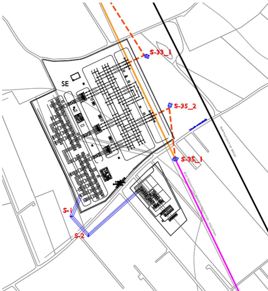
Figura 2: Layout Stazione elettrica e Cabina Primaria
