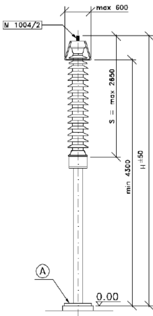
Figura 17: Scaricatore
