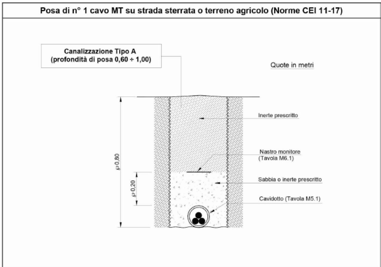
Figura 8: Modalità di posa su strada sterrata/asfaltati
