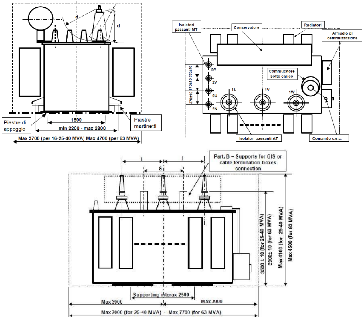
Figura 15: Trasformatore AT/MT - Schemi costruttivi
