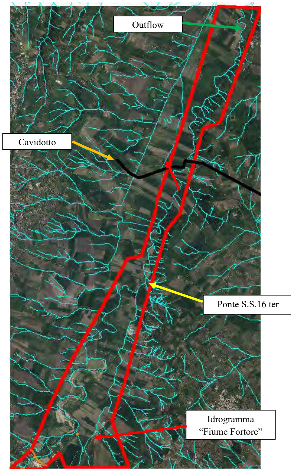
Figura 5.6.1: Dominio di calcolo del modello Fortore
