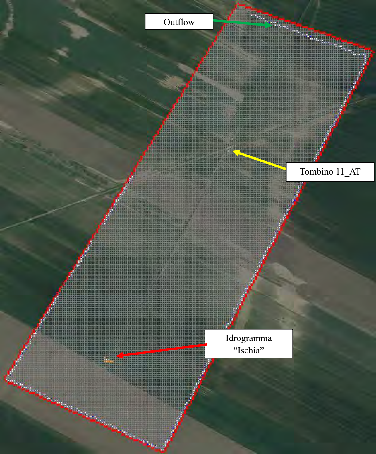
Figura 5.7.1: Dominio di calcolo del modello C
