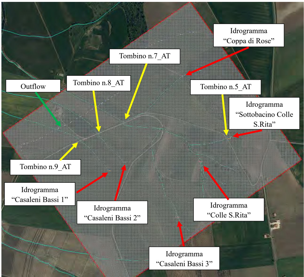
Figura 5.5.1: Dominio di calcolo del modello B
