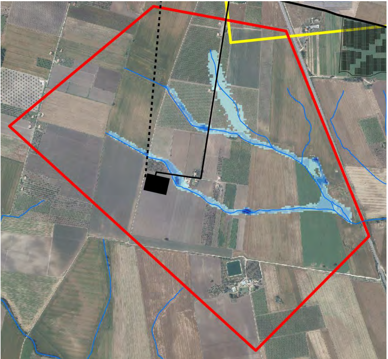
Figura 5.1.1.1: Aree inondabili per T=200anni del modello n.2
