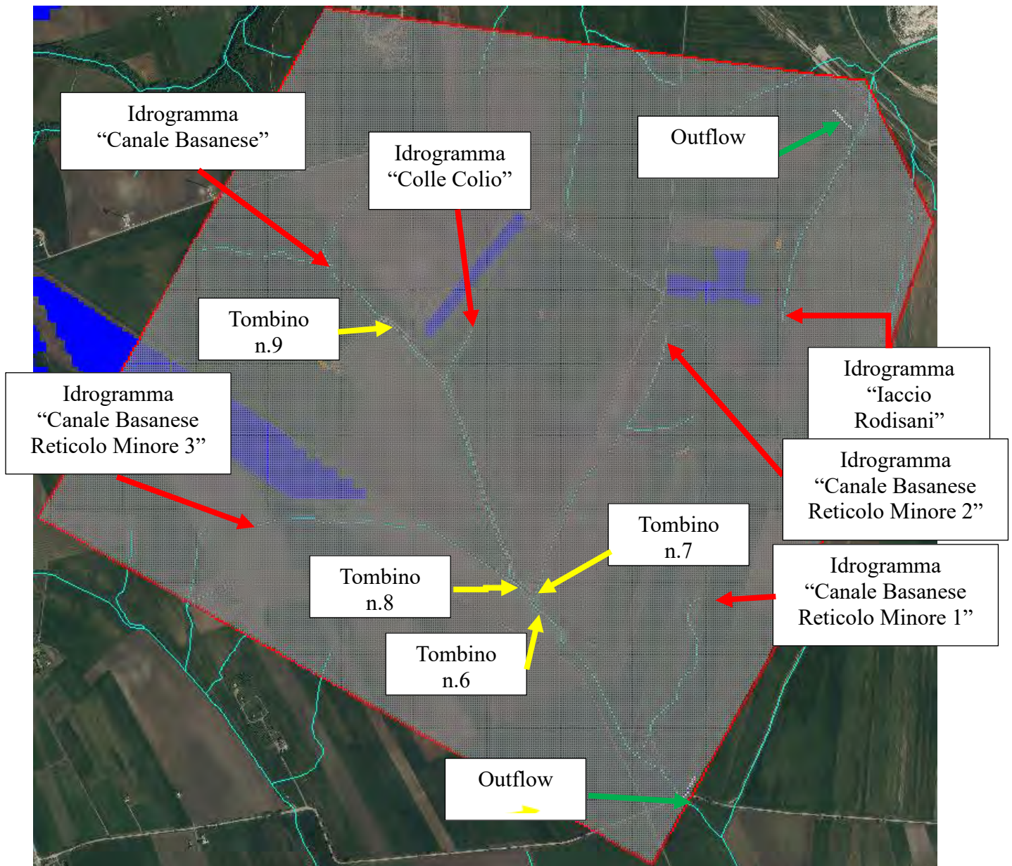
Figura 5.2.1: Dominio di calcolo del modello n.3
