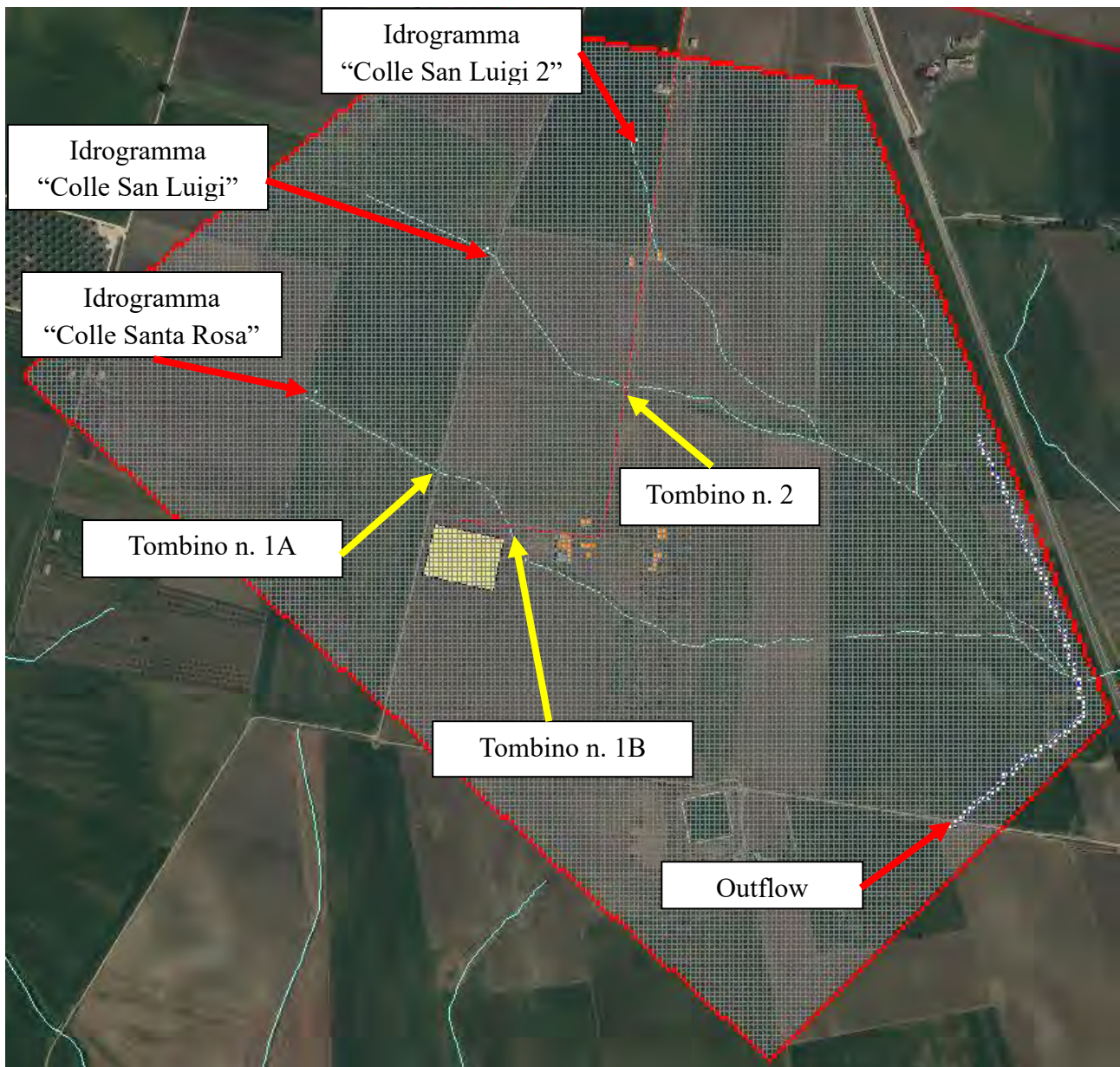
Figura 5.1.1: Dominio di calcolo del modello n.2
