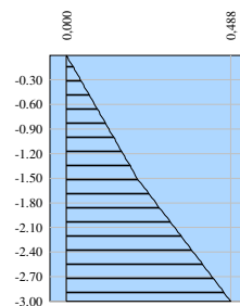
Pressione verticale [Portanza di punta]
