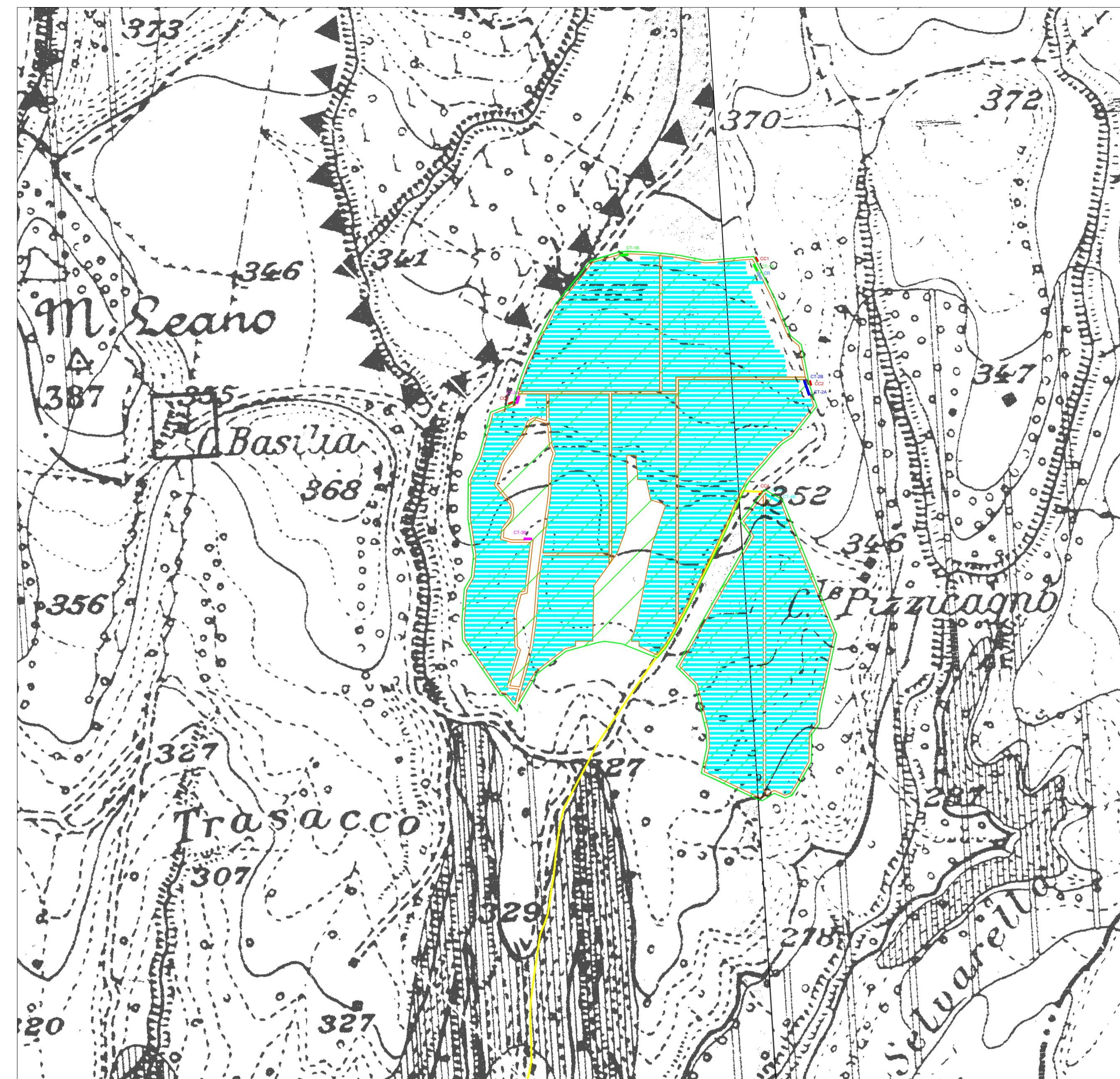
Layout impianto FV su Piano Regolatore del Comune di Viterbo - scala 1:5000
