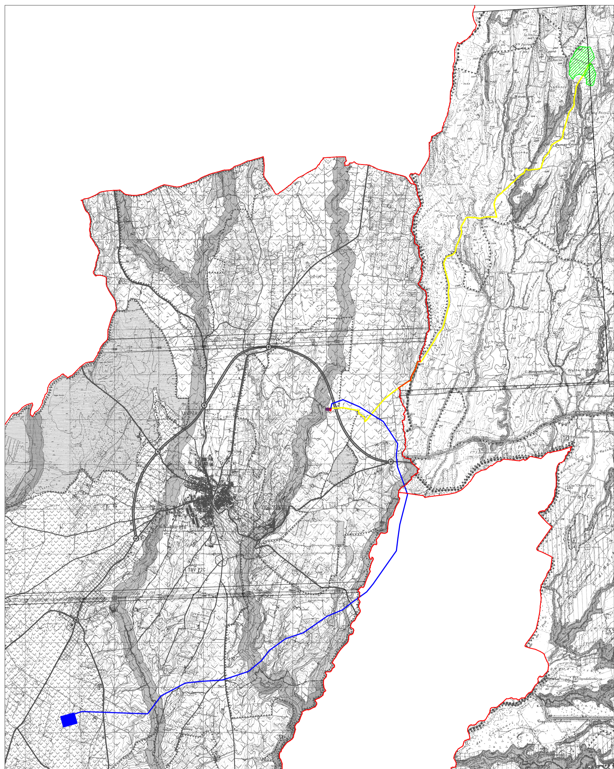
Layout impianto FV su Piano Regolatore del Comune di Tuscania - scala 1:5000
