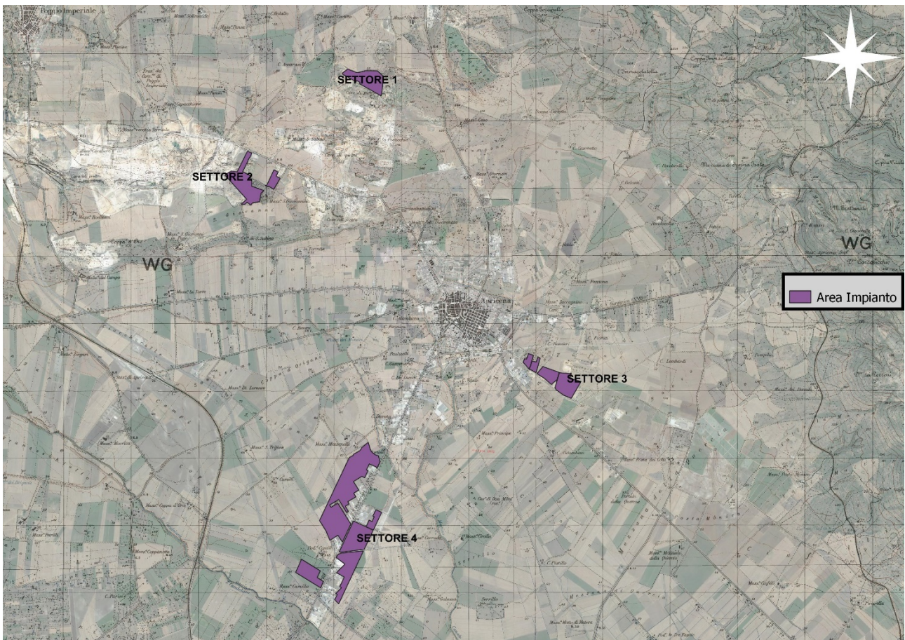
Figura 1- Veduta aerea di dove verrà posizionato Impianto Fotovoltaico
