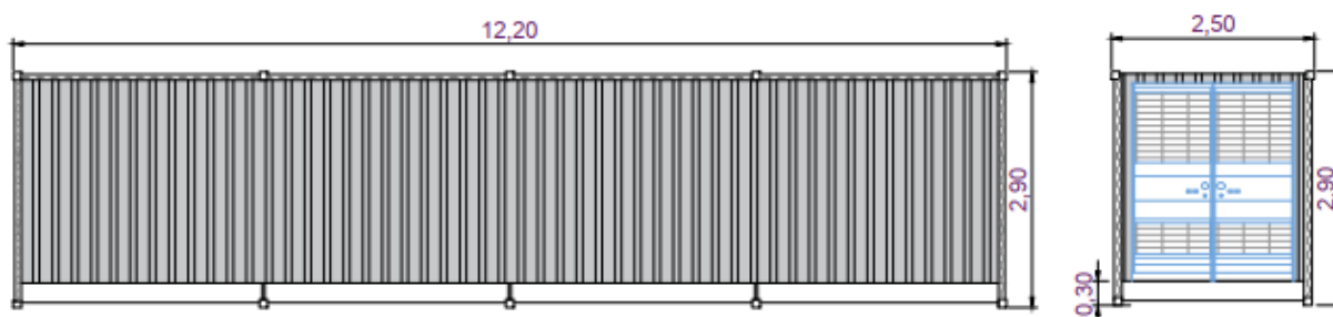
Figura 7-12 – Layout tipico Modulo batterie
