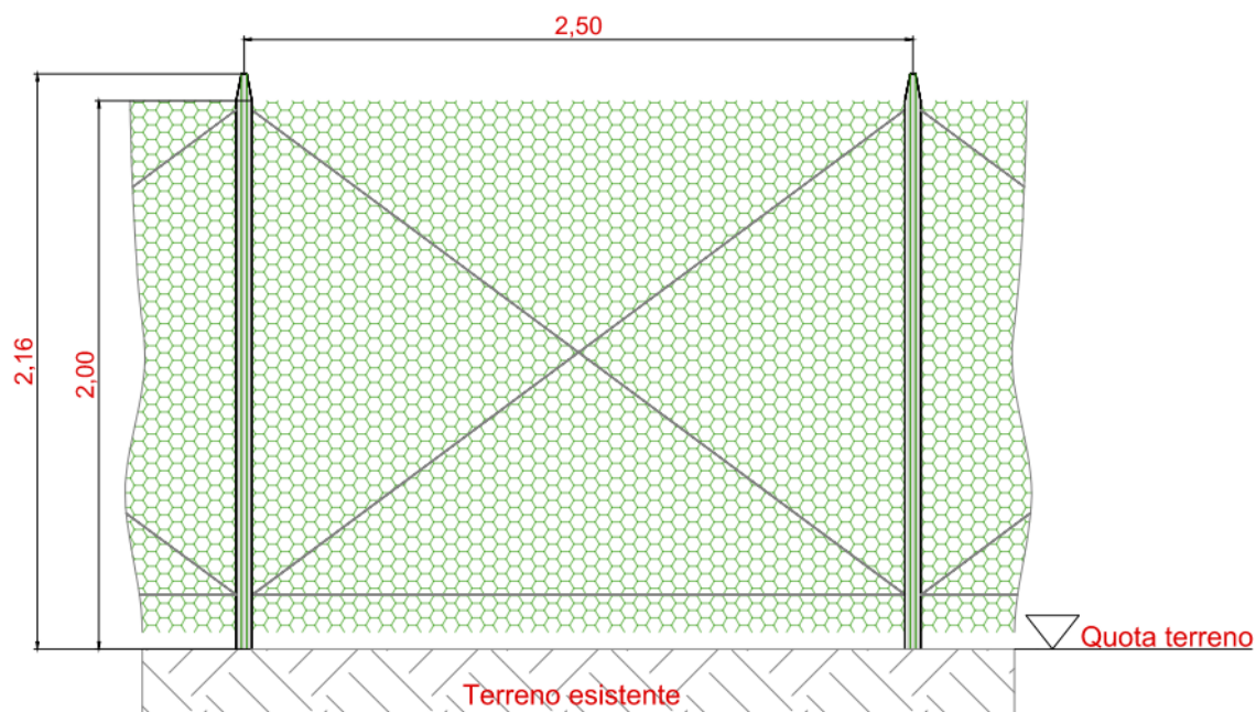
Figura 8-1 – Tipologia tipica recinzione
