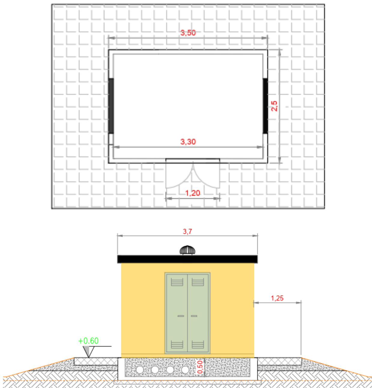
Figura 7-6 – Layout tipico Cabina servizi ausiliari
