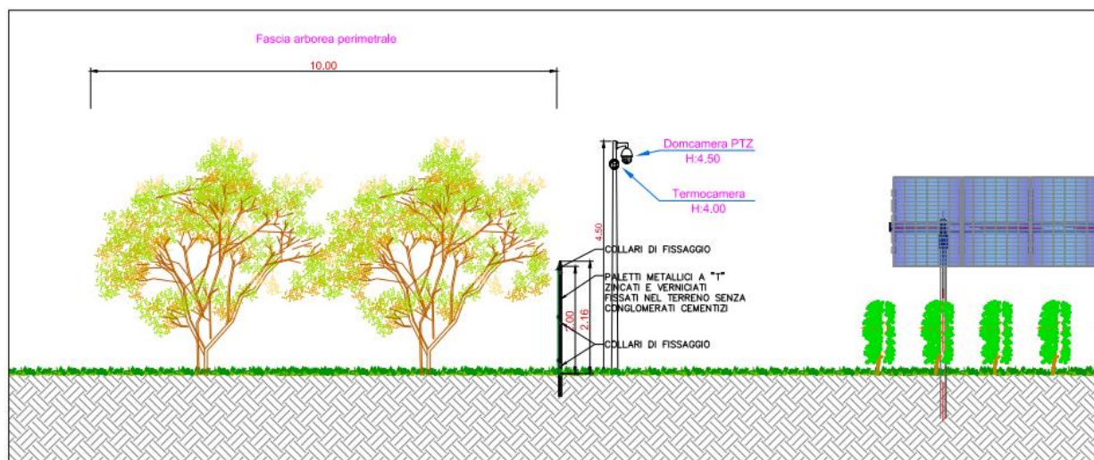
Figura 8-5 – Sezione fascia arborea perimetrale esterna alla recinzione
