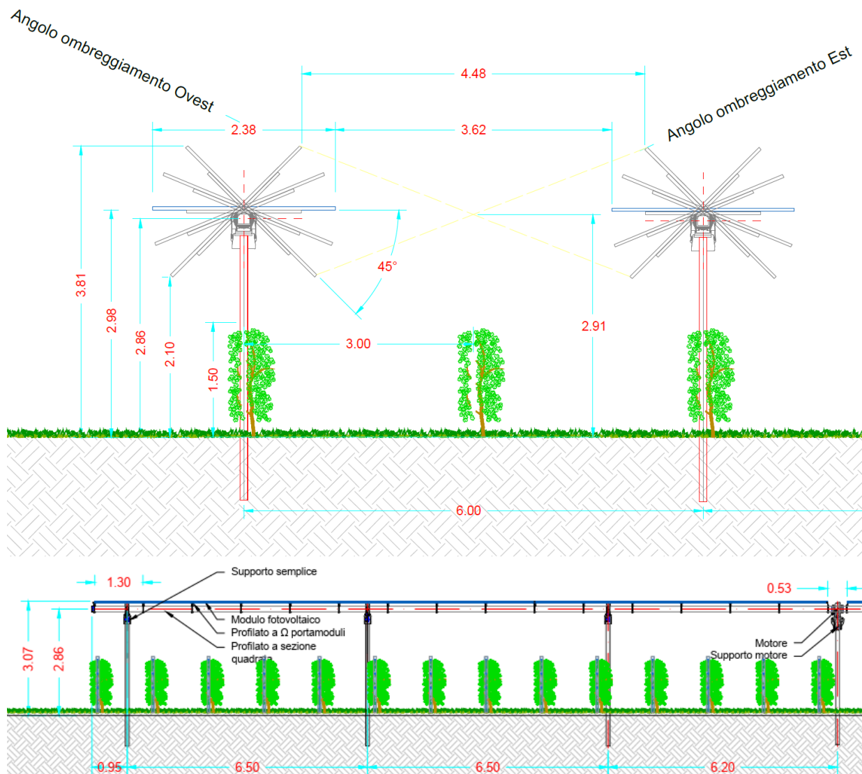
Figura 7-3 – Sezione trasversale tipologica struttura Tracker
