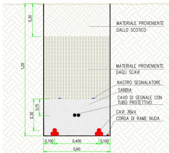
Figura 8-8 – Sezione tipica posa cavi 30 kV
