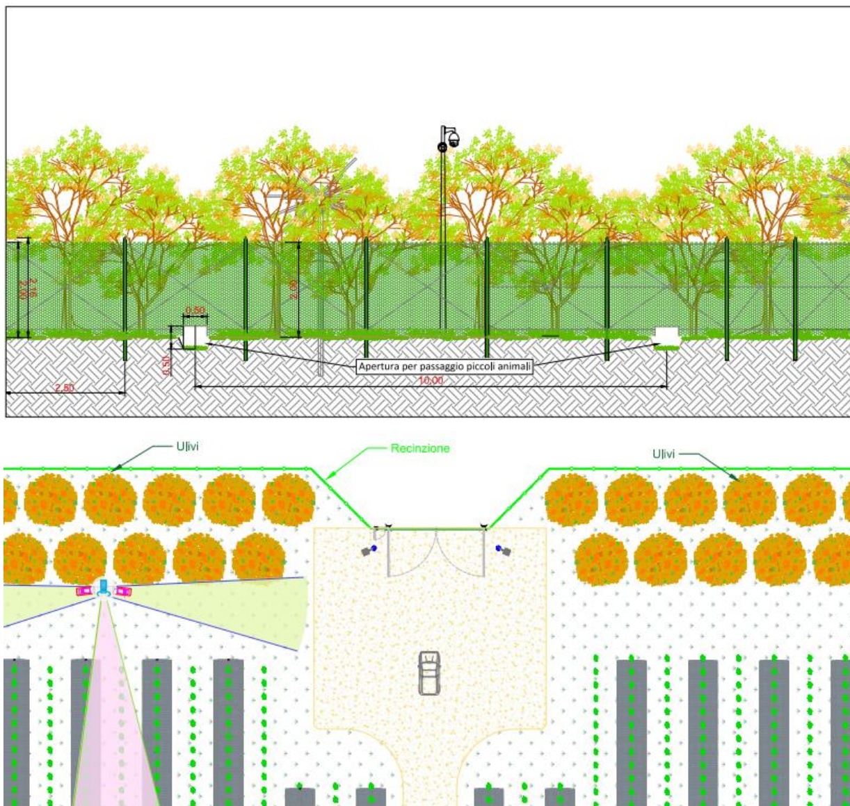
Figura 8-4 – Sezione fascia arborea perimetrale interna alla recinzione
