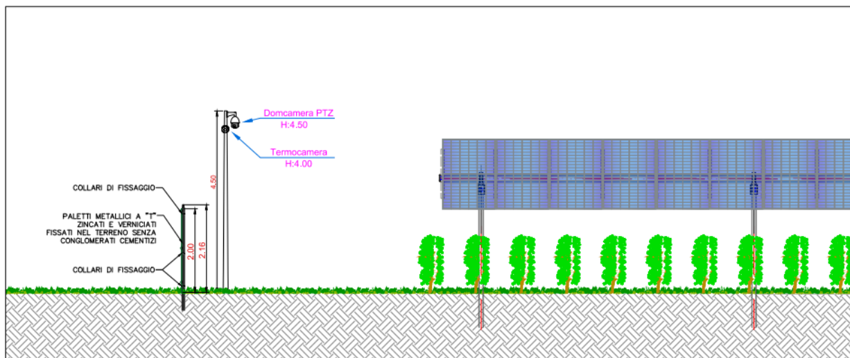
Figura 8-6 – Sezione recinzione senza fascia arborea
