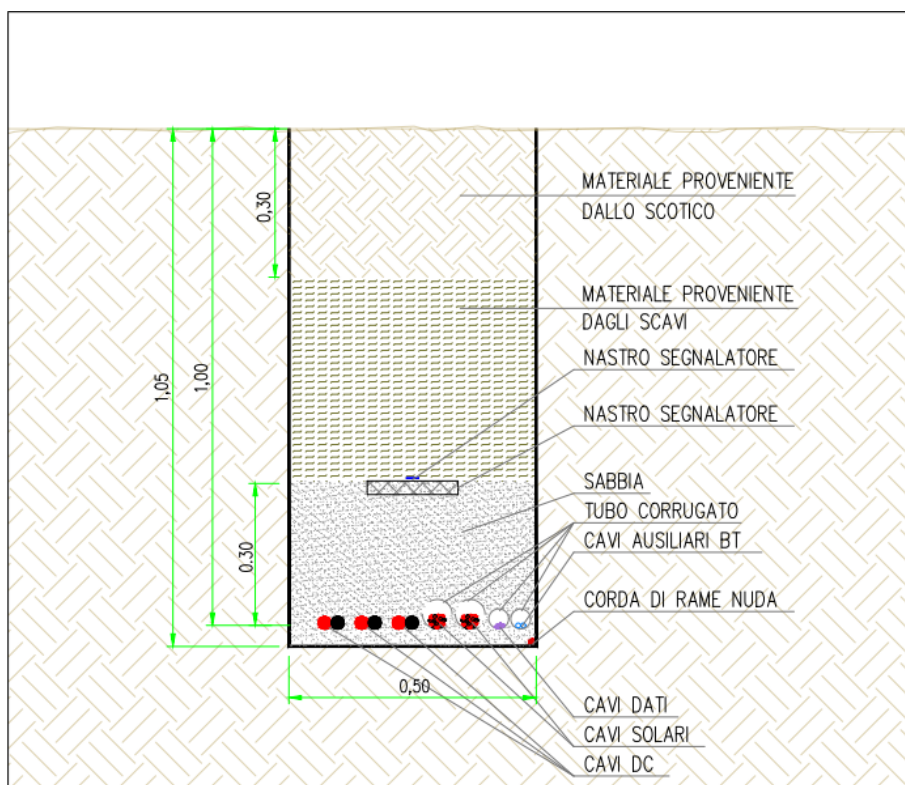
Figura 8-7 – Sezioni tipiche posa cavi BT
