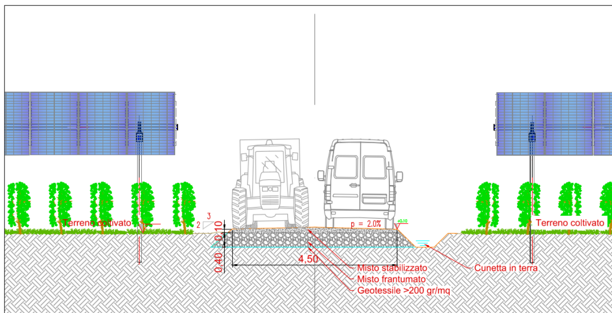
Figura 8-2 – Sezione tipica strada interna con cunetta
