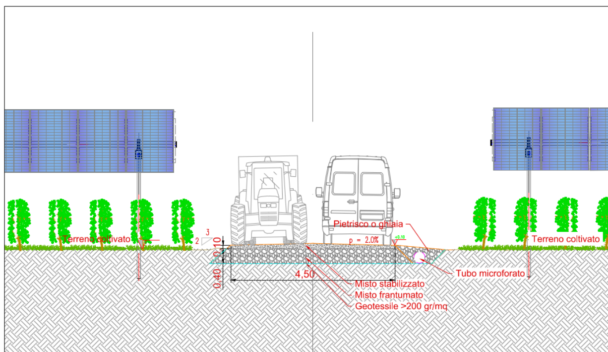
Figura 8-3 – Sezione tipica strada interna con drenaggio
