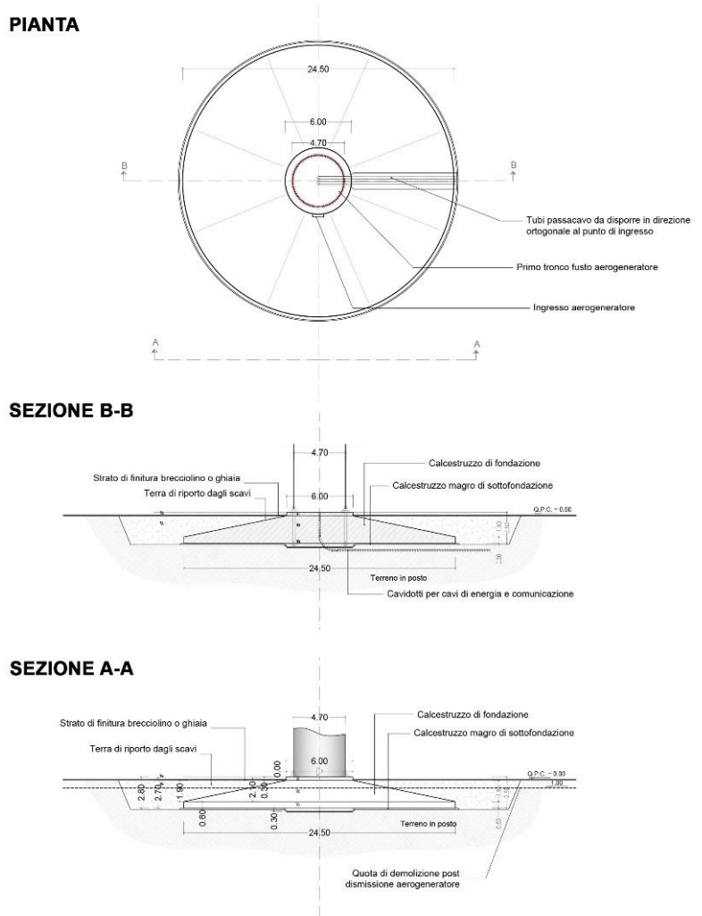
Figura 1 – Pianta e vista della fondazione tipo dell'aerogeneratore
