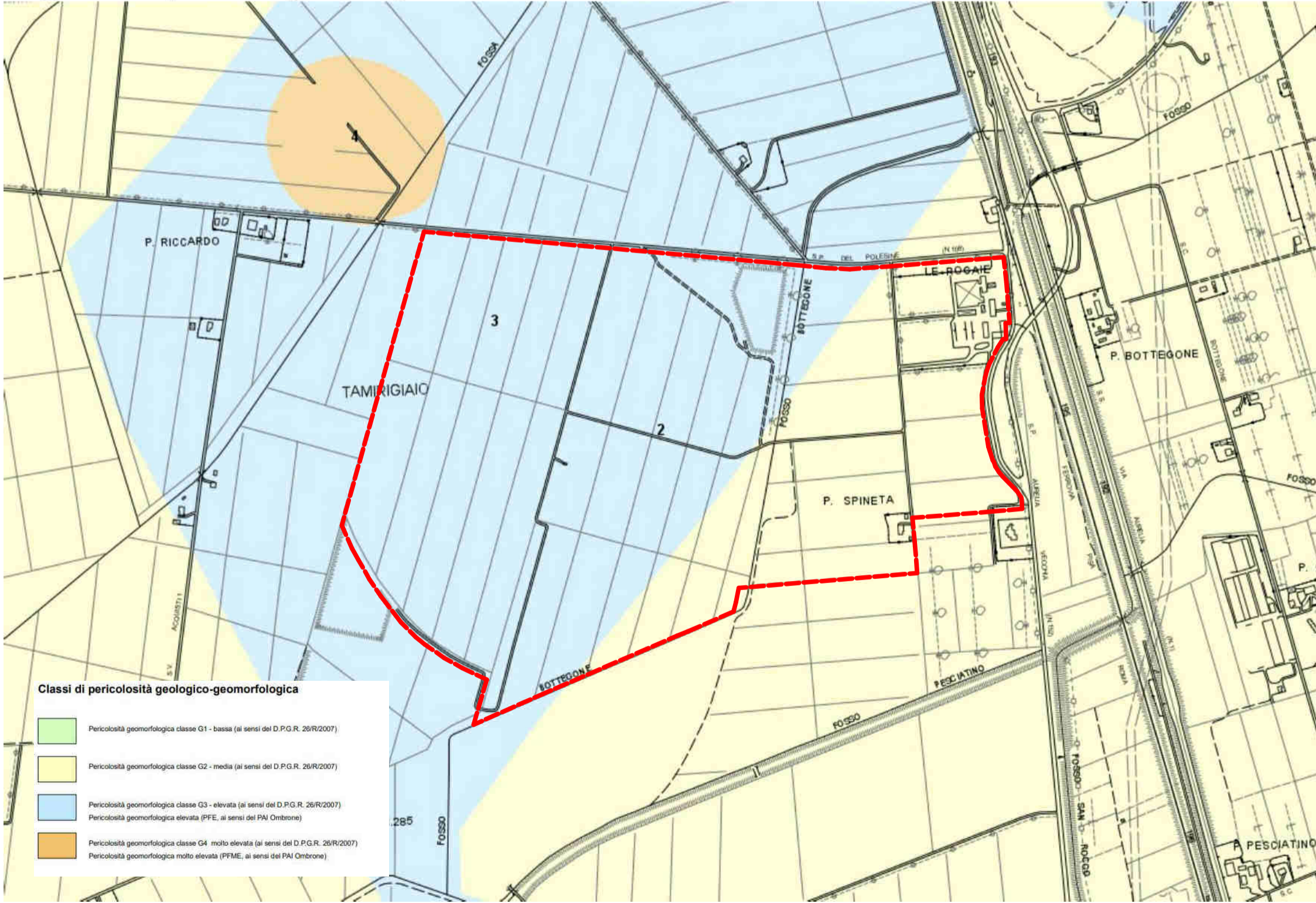
RU GROSSETO_Carta della pericolosità geomorfologica
