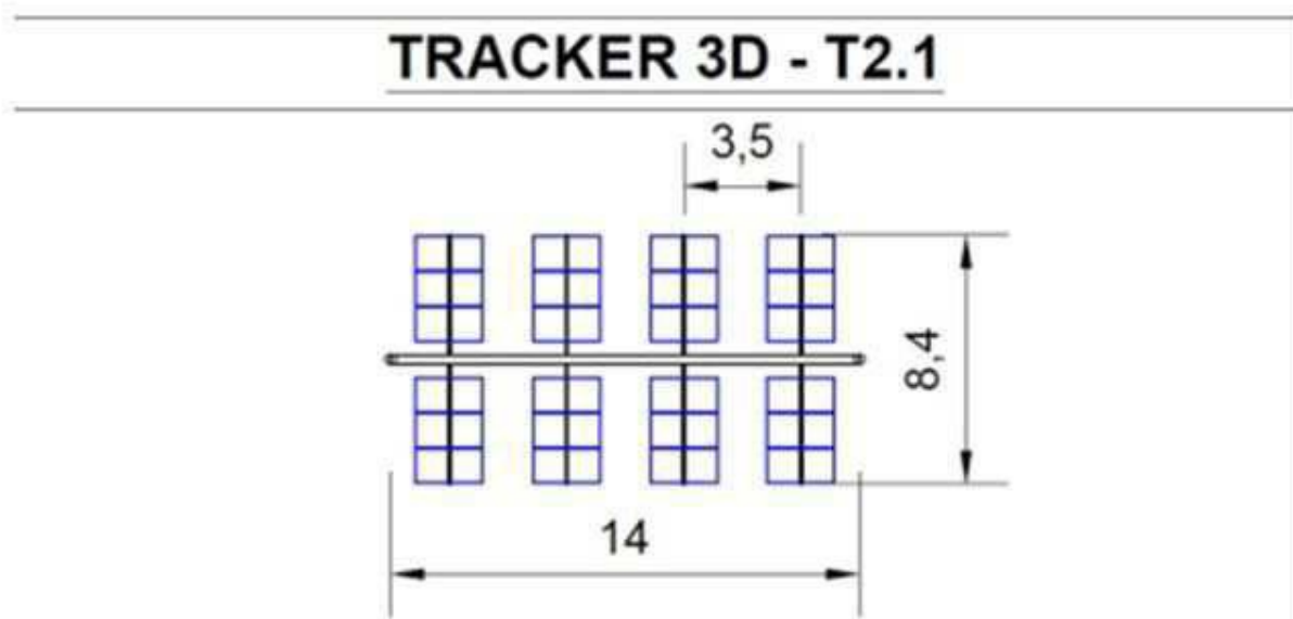
Figura 37-Tipologia di tracker
