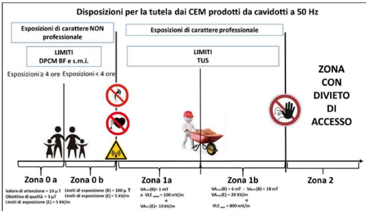
Figura 6: Misure di prevenzione e protezione per la tutela dai CEM prodotti da cavidotti a 50 Hz
