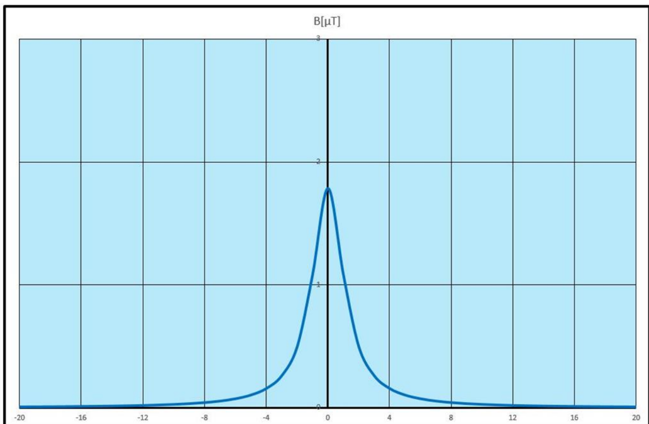
Figura 5: Induzione magnetica generata durante l'esercizio dalle linee elettriche MT valutata ai sensi della Norma CEI 211-4 – Guida ai metodi di calcolo dei campi elettrici e magnetici generati da linee elettriche. Fasi disposte a trifoglio, profondità di posa 1,20 m.
