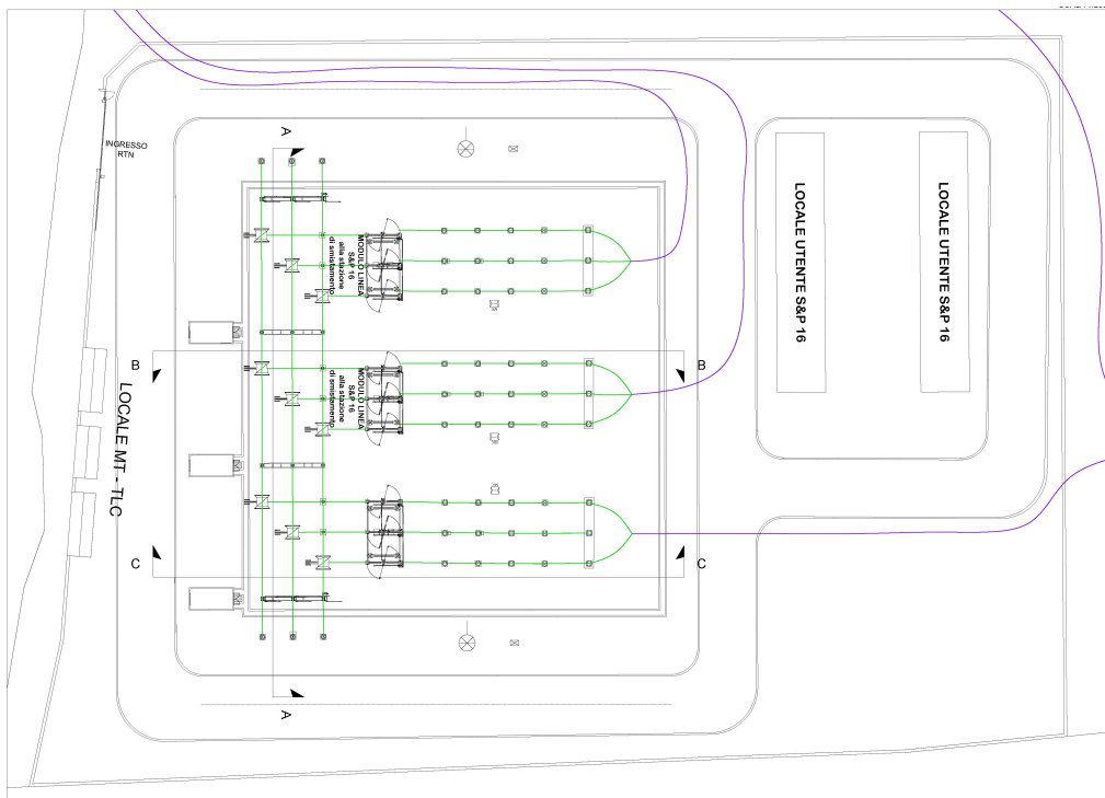
FIGURA . Pianta elettromeccanica generale – STAZIONE UTENTE
