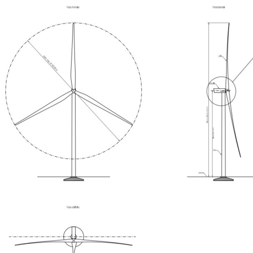
Figura 7 – Pianta e prospetti aerogeneratore
