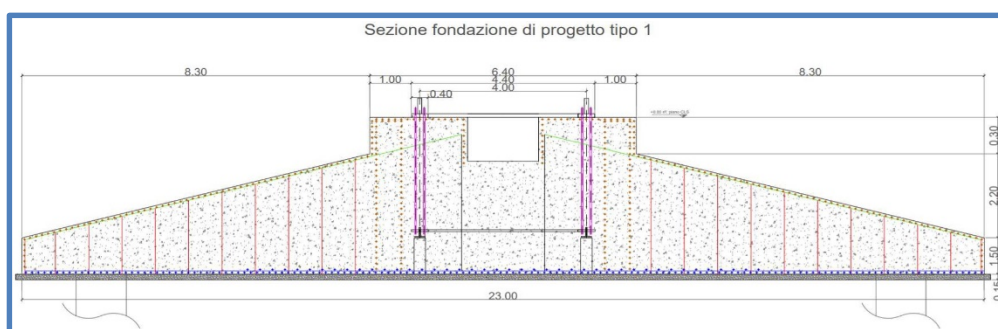
Figura 8 - Tipologia fondazione
