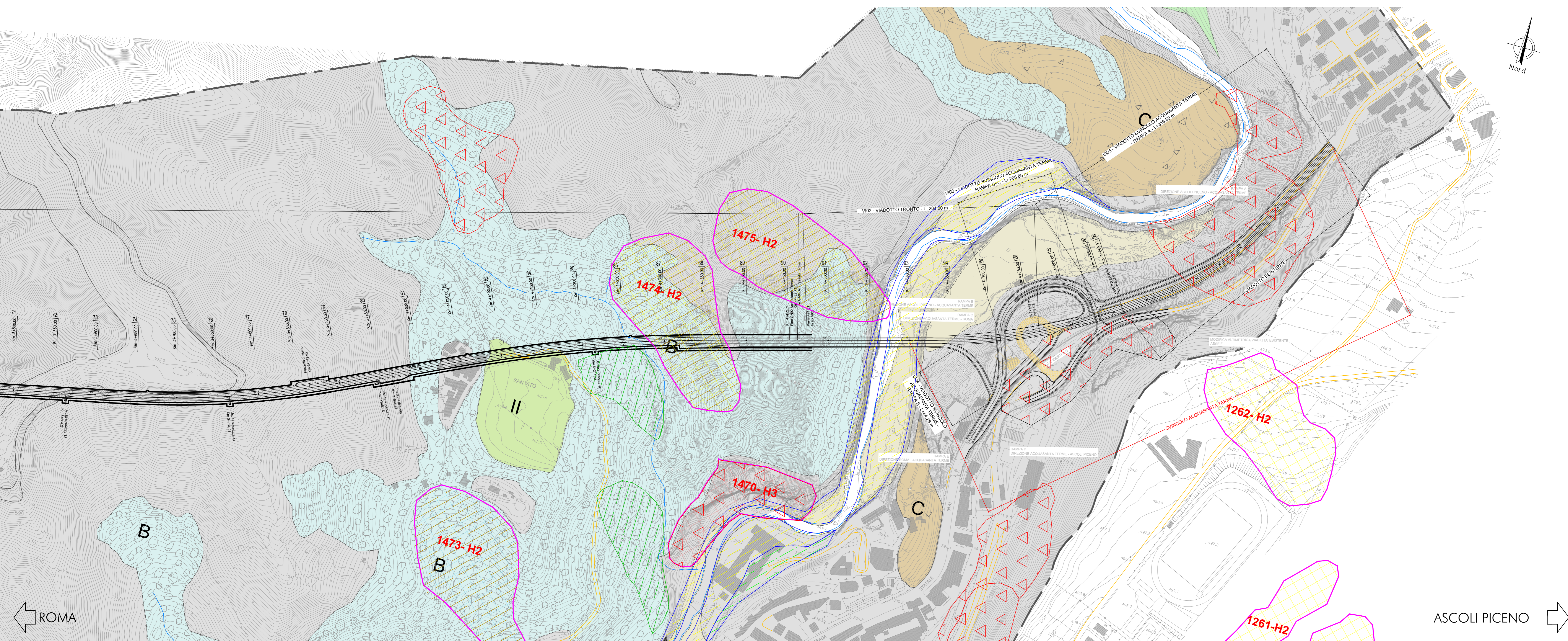
PLANIMETRIA SCALA 1:2000
