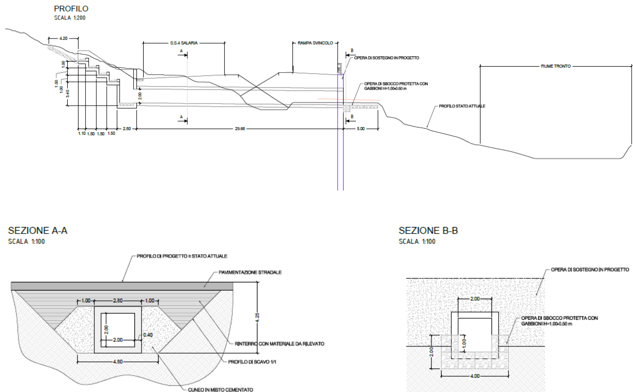
Figura 2.7: Profilo e sezione tipo tombino scatolare
