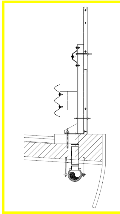
Figura 2.13: Sezione tipo in viadotto.
