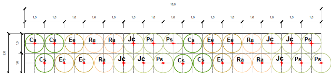
Figura 2.37: Planimetria del sesto d’impianto del MODULO F
