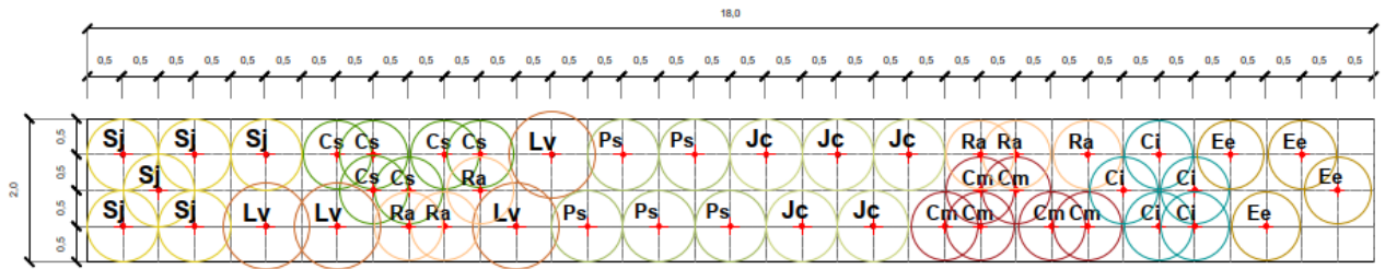
Figura 2.28: Planimetria sesto d'impianto MODULO C
