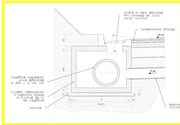
Figura 2.12: Sezione in corrispondenza del pozzetto.
