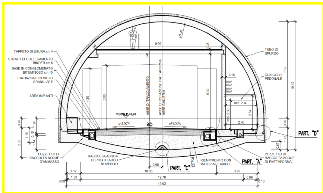
Figura 2.14: Sezione tipo idraulica di piattaforma in galleria.
