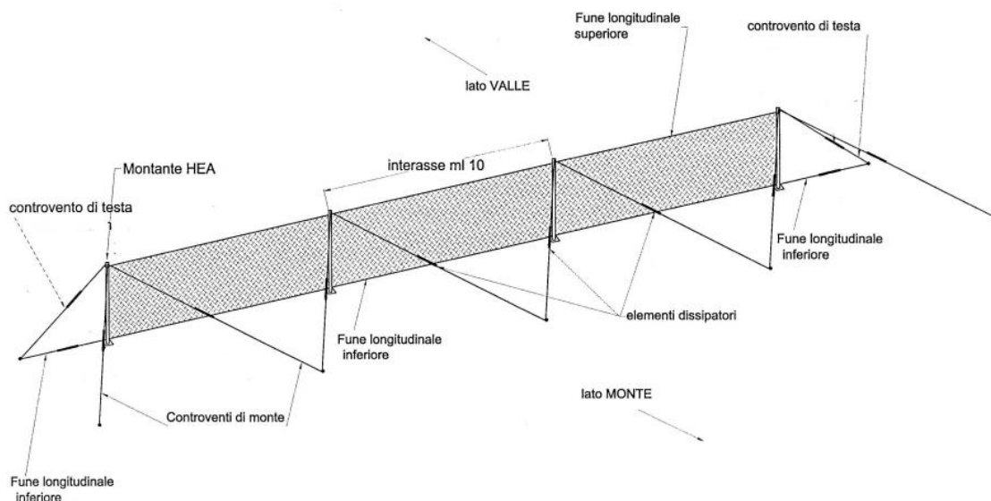
Figura 2.44: Schema assonometrico tipologico della barriera paramassi.
