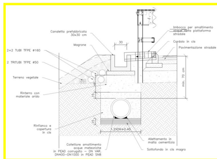
Figura 2.9: Schema drenaggio rilevato.
