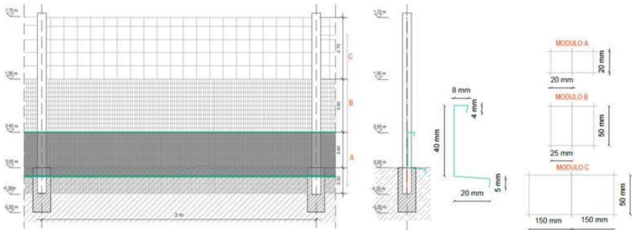
Figura 2.41: Rete antiattraversamento fauna
