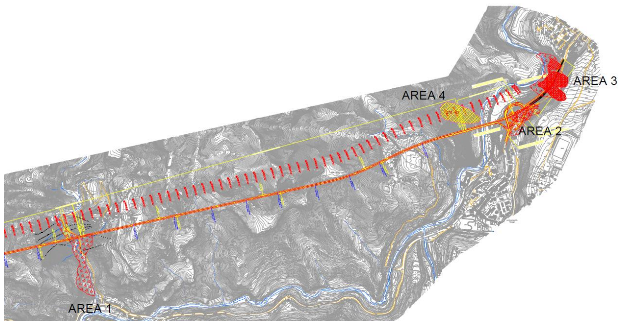
Figura 2.8 - Planimetria frane interferenti con l’opera.
