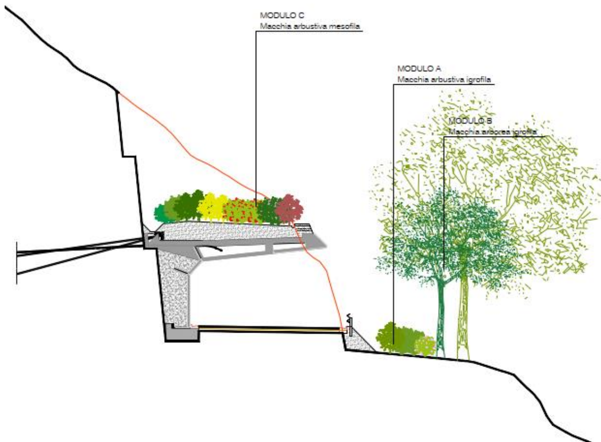
Figura 2.45: Sezione barriera paramassi con nuovo impianto arbustivo di mitigazione
