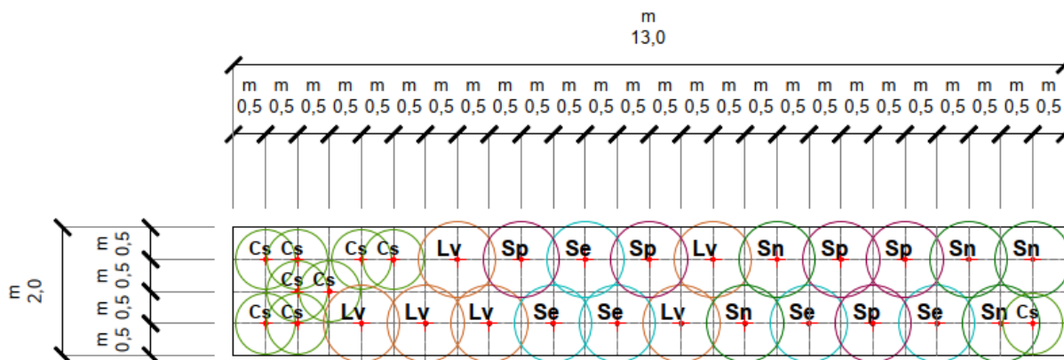
Figura 2.22: Planimetria sesto di impianto MODULO A
