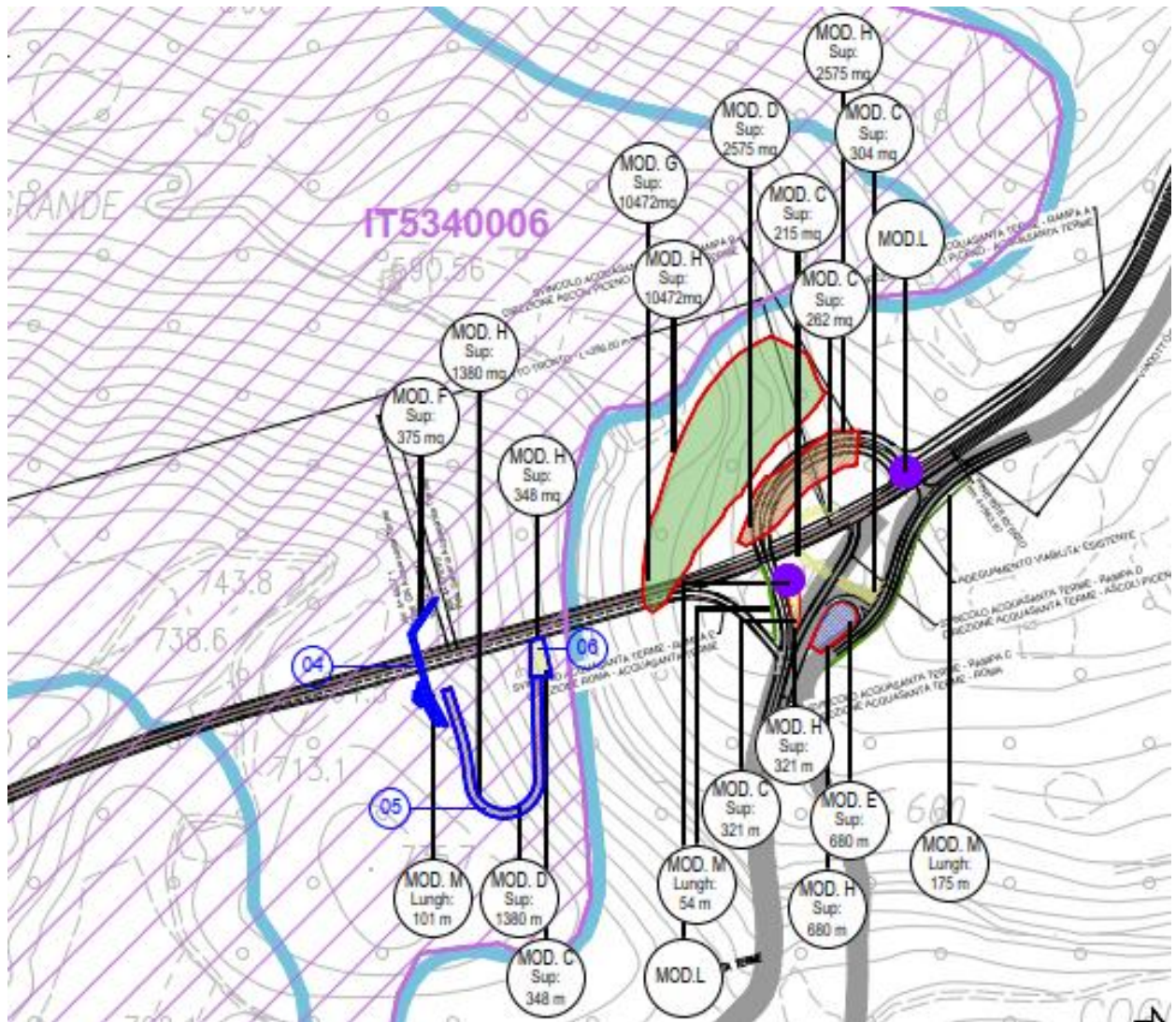
Figura 2.48: Area per la compensazione dei siti natura 2000 - aree 04, 05 e 06
