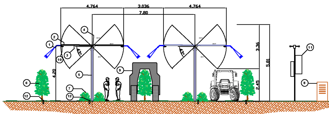
Schema TRAKER Tipologia impianto AFV
