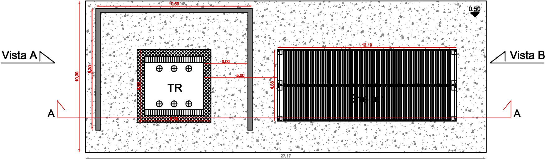
Pianta
