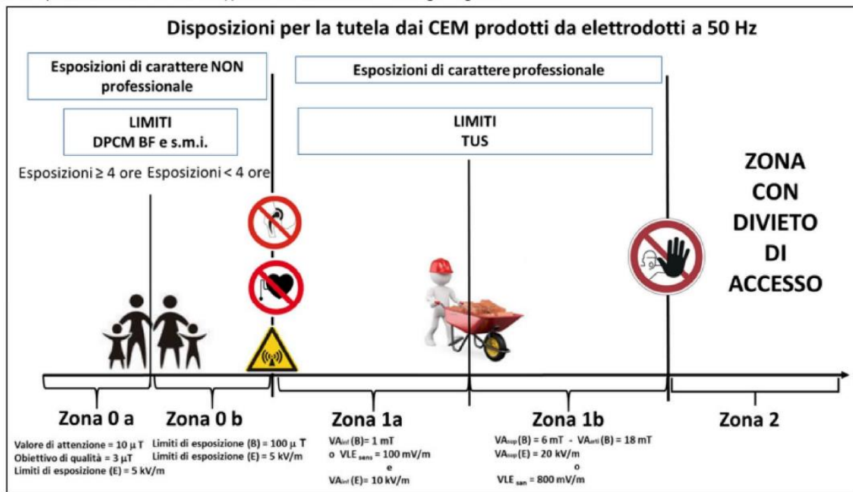
Figura 10: Misure di prevenzione e protezione per la tutela dai CEM prodotti da Elettrodotti a 50 Hz
