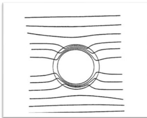
Figura 17: andamento qualitativo della deformazione delle linee di forza di un campo magnetico uniforme per effetto di un nucleo in materiale ferromagnetico
