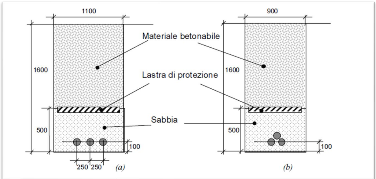
Figura 18: schermatura cavi elettrici interrati
