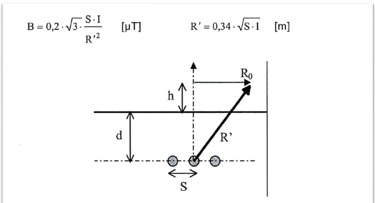
Figura 8: Schema di principio per il calcolo delle distanze da terne di cavi interrati con posa in piano/sbarre AT isolate in aria oltre le quali l'induzione magnetica è inferiore all'obiettivo di qualità – Norma CEI 106-11 – Guida per la determinazione delle fasce di rispetto per gli elettrodotti secondo le disposizioni del DPCM 8 luglio 2003
