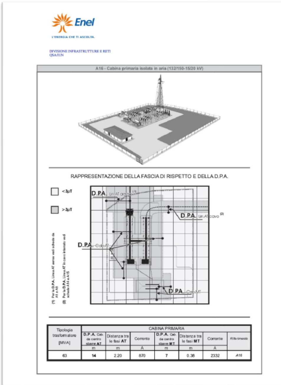
Figura 7: DPA Cabina Primaria AT/MT Enel equipaggiata con n° 2 trasformatori AT/MT da 63 MVA- Linea Guida per l'applicazione del § 5.1.3 dell'Allegato al D.M. 29.05.08 – Distanza di prima approssimazione da linee e cabine elettriche
