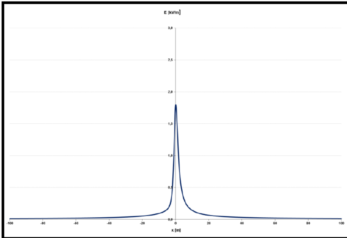
Figura 11: Campo elettrico generato dalla Linea durante l'esercizio valutato applicando la procedura della Norma CEI 211-4 - Guida ai metodi di calcolo dei campi elettrici e magnetici generati da linee elettriche
