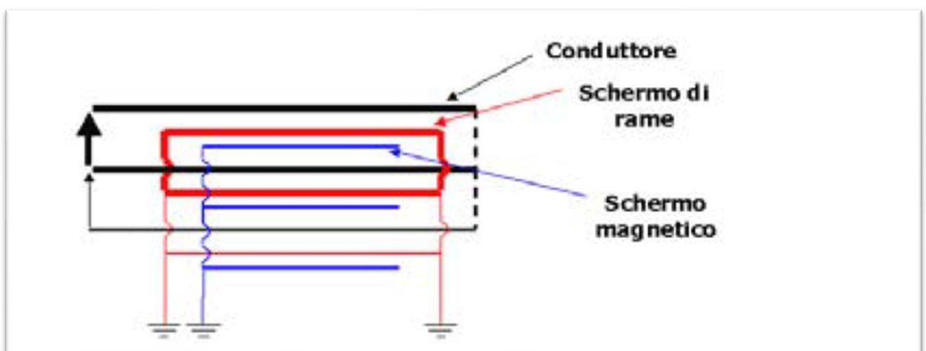
Figura 19: schema bidimensionale del cavo unipolare e della messa a terra degli schermi- tecnica "solid bonding"
