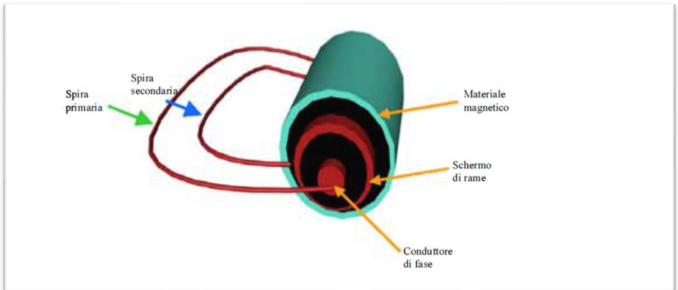
Figura 20: schema tridimensionale del cavo a debole emissione di campo magnetico- tecnica "Solid-bonding"
