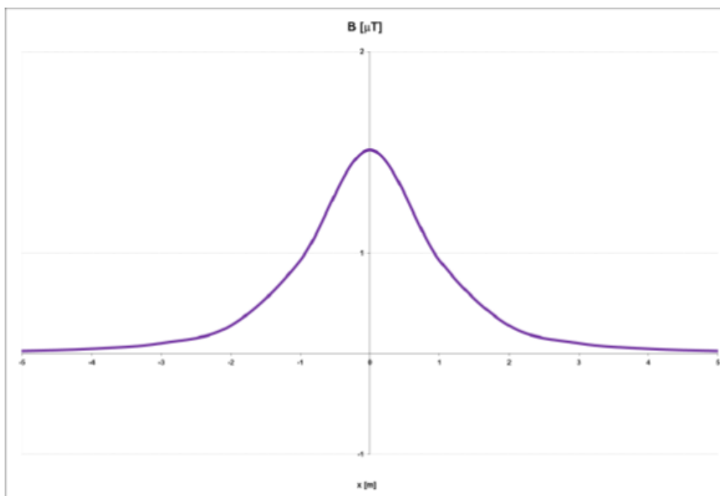
Figura 5: Induzione magnetica generata durante l'esercizio valutata ai sensi della Norma CEI 211-4 – Guida ai metodi di calcolo dei campi elettrici e magnetici generati da linee elettriche
