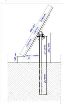
Vista laterale - Tilt massimo
