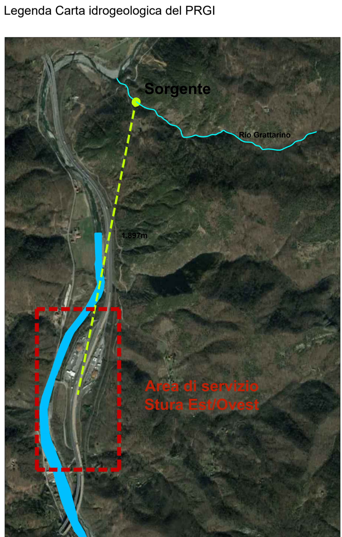
Individuazione sorgente più prossima (Rio Grattarino) Stralcio Carta idrogeologica del PRGI Comune di Belforte, Monferrato
