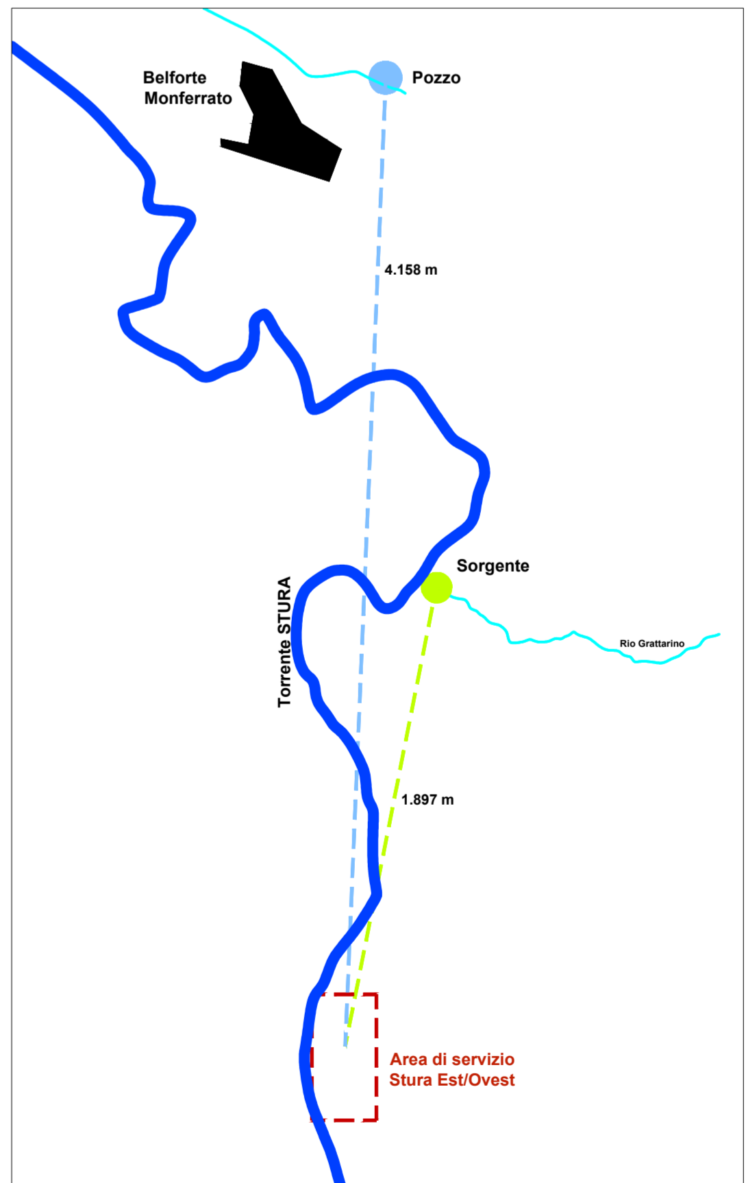
Individuazione Torrente Stura e pozzo più prossimo Stralcio Carta idrogeologica del PRGI Comune di Belforte, Monferrato
