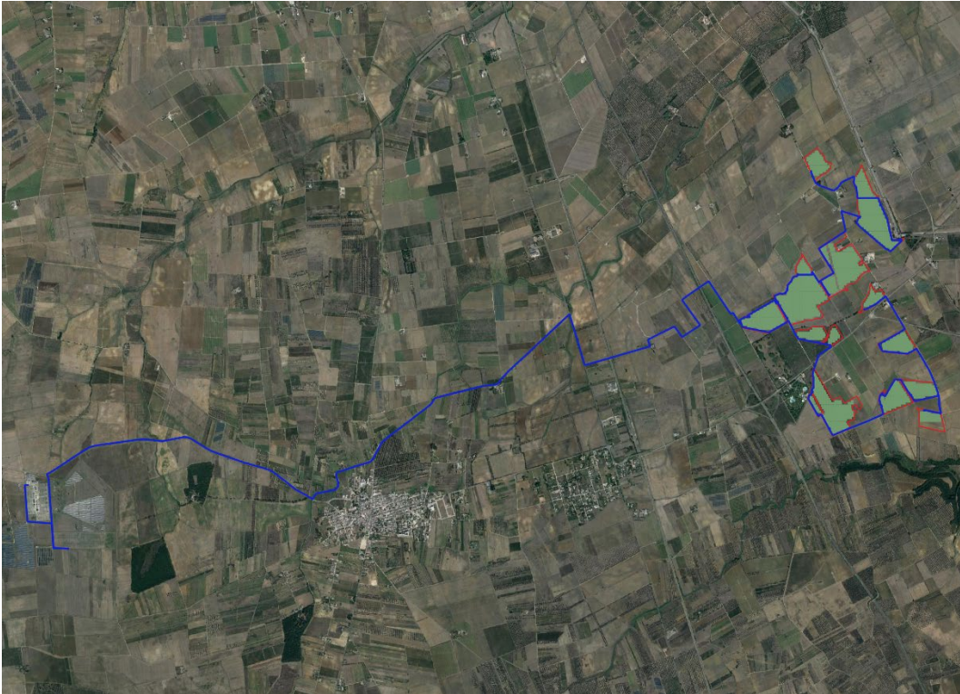
Tavola n. 14: layout dell’impianto su ortofoto
