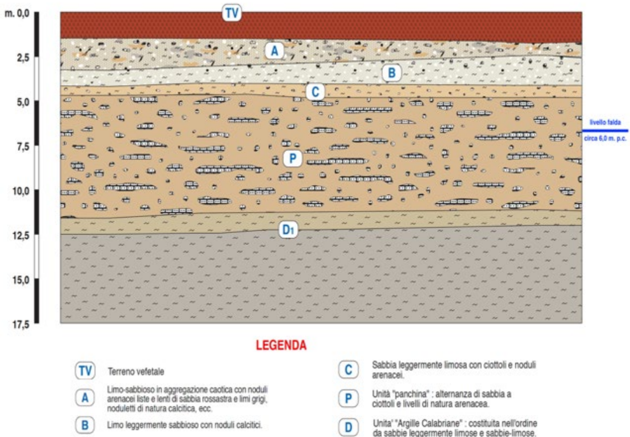
Tavola n. 47: rappresentazione stratigrafica tipica dell'area della "Conca di Brindisi".
