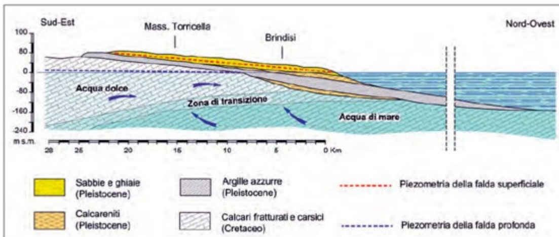
Tavola n. 48: schema idrico, sotterraneo: artesiano e freatico.
