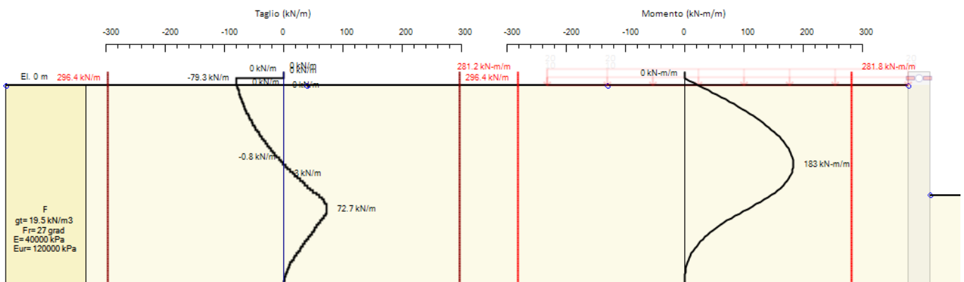
Fig. 8: Sollecitazioni e verifiche strutturali (A1+M1+R1)
