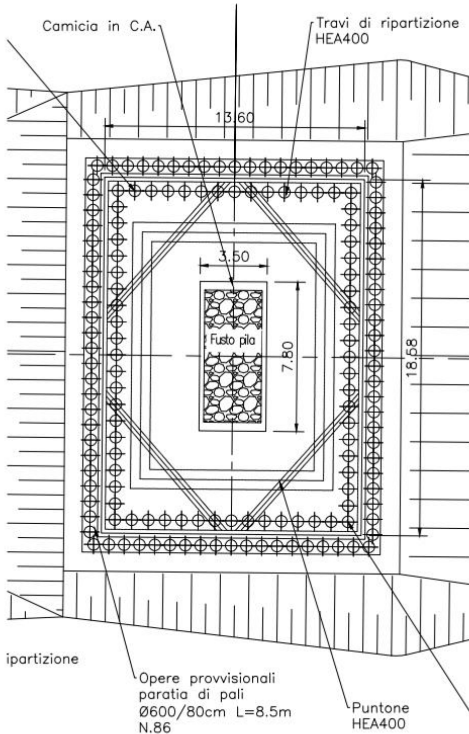
Fig. 2 Vista in pianta
