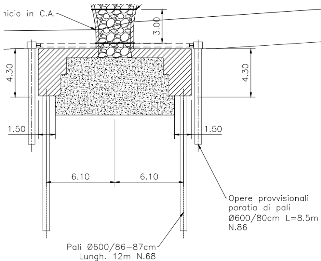
Fig. 1 – Sezione trasversale
