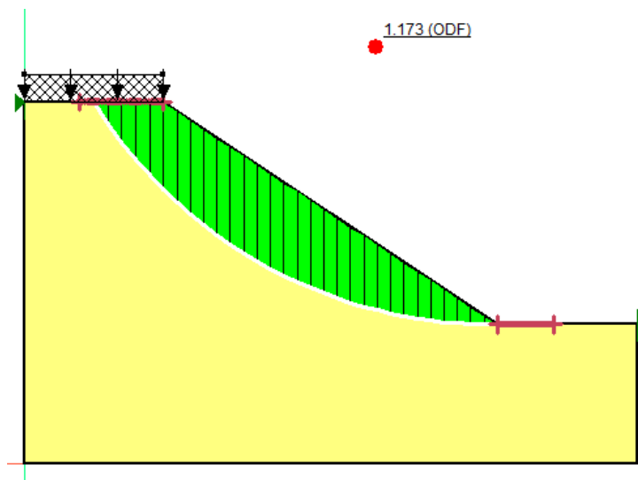
Fig. 10 –Verifica stabilità scavo
