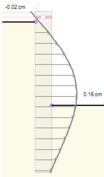
Fig. 9 –Diagramma degli spostamenti orizzontali allo SLE
