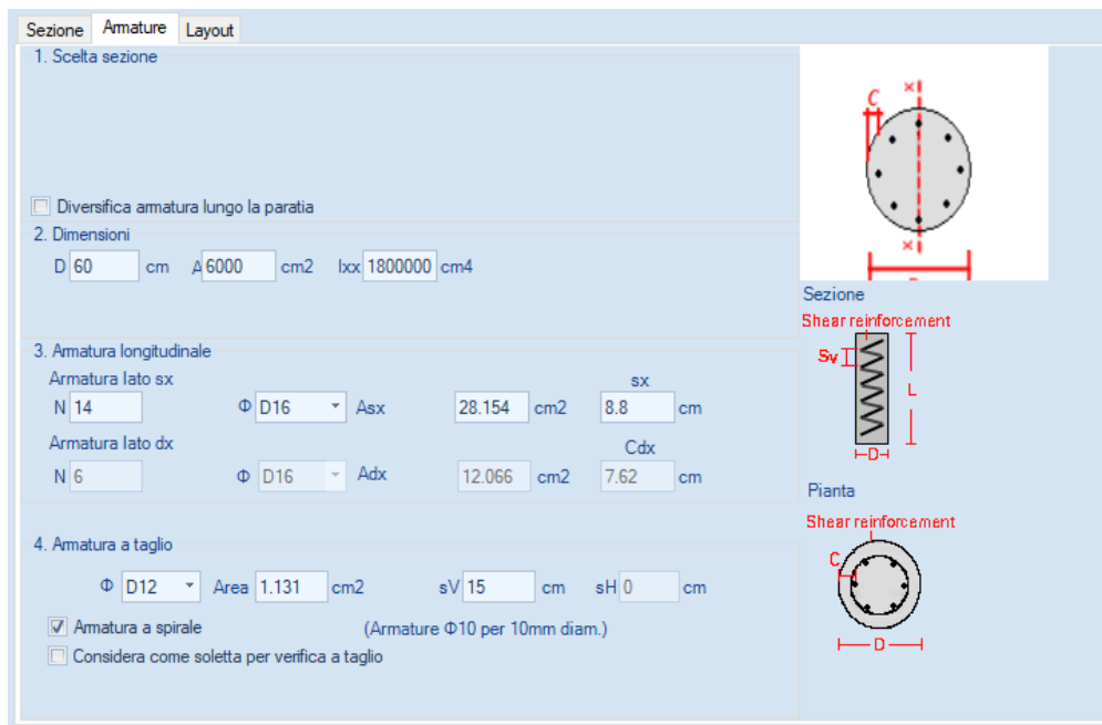
Fig. 7: Armature longitudinali e trasversali dei pali
