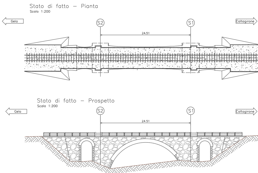
Figura 1: Ricostruzione carpenteria opera;
