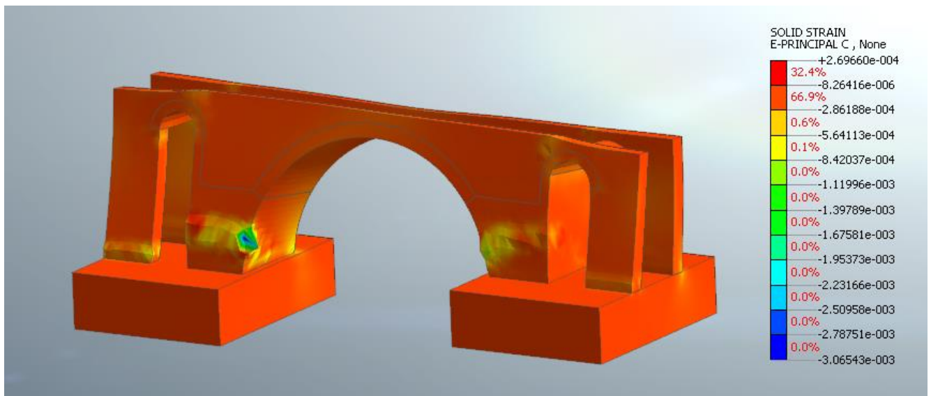
Figura 38: Deformazione E3 (principale di compressione) allo step di collasso
