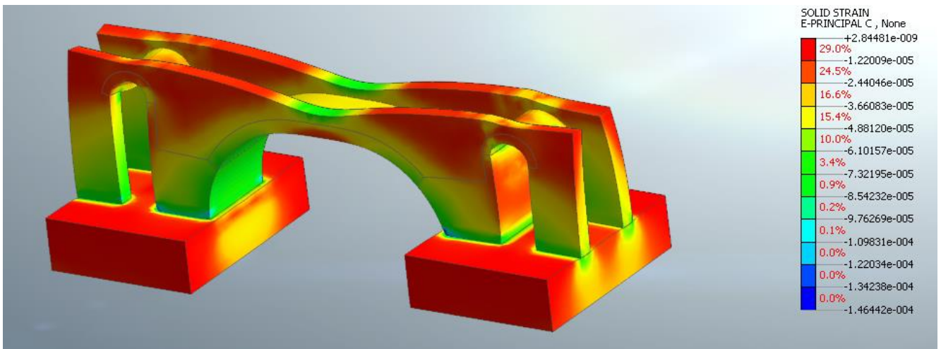
Figura 16: deformazioni massime di compressione (moltiplicatore del carico pari a 1)
