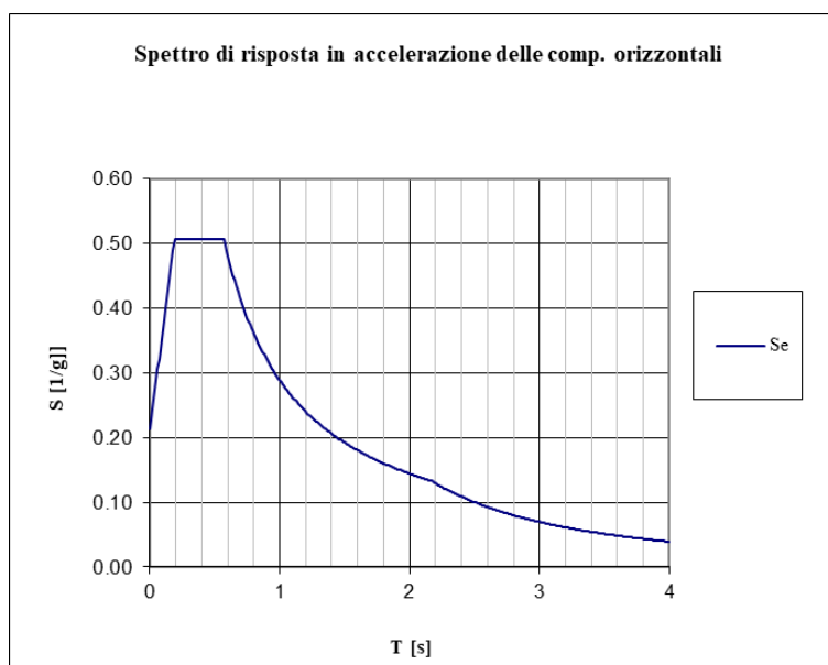
Figura 9: Spettro accelerazioni orizzontali
