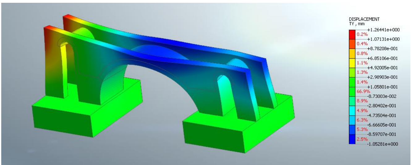
Figura 21: 2° Modo di vibrare - secondo modo in direzione trasversale
