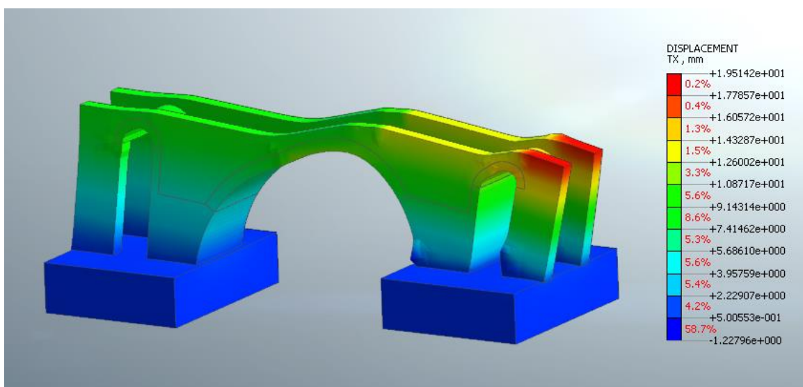
Figura 30: Mappa cromatica spostamento DX step di collasso
