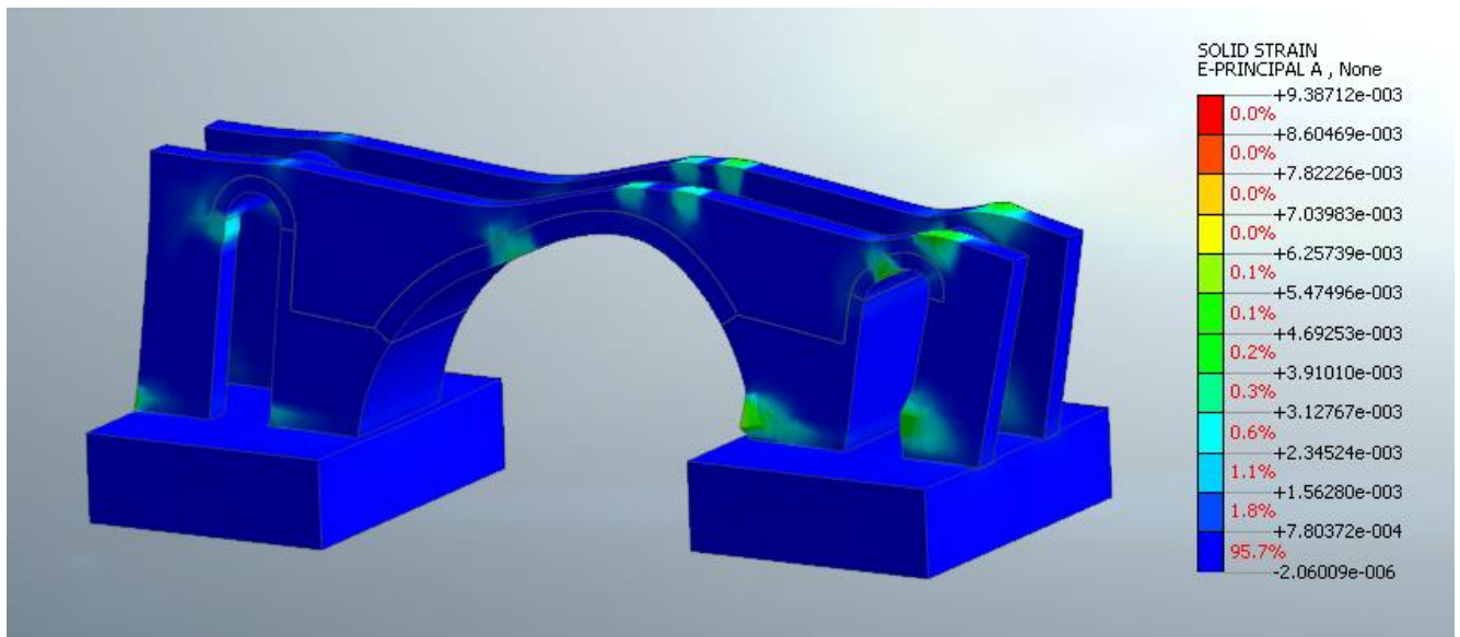
Figura 31: Deformazione E1 (principale di trazione) allo step collasso
