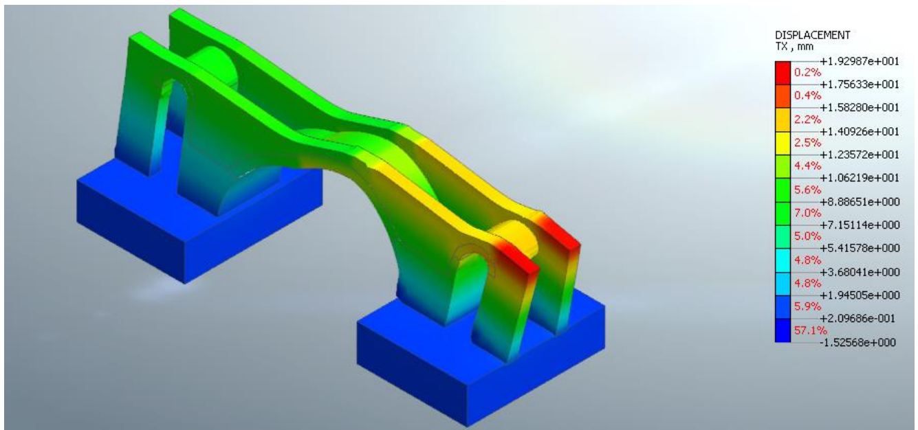
Figura 24: Mappa cromatica spostamento in direzione X allo step di collasso
