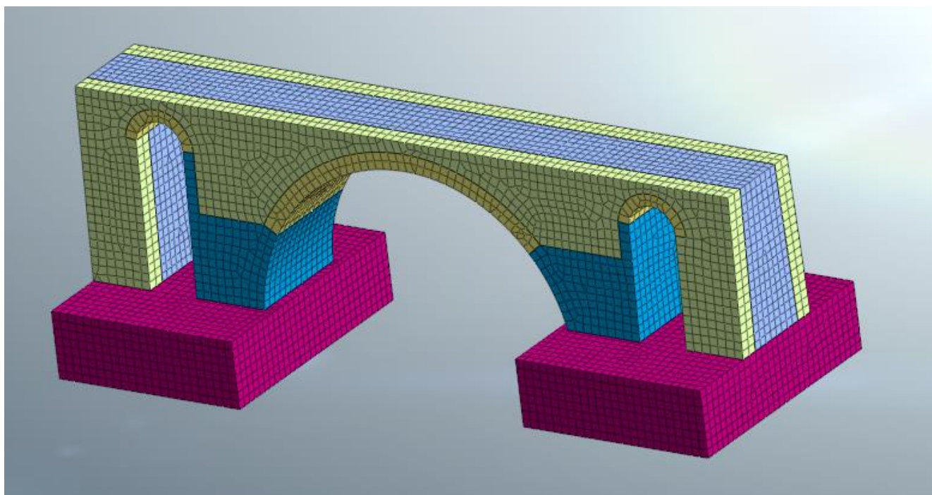
Figura 8: Modello dell'opera completo
