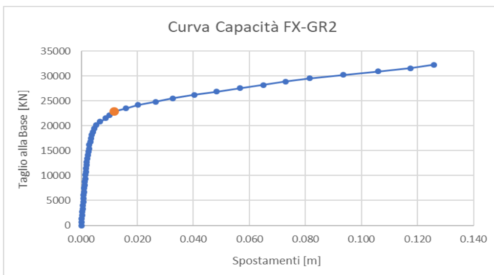
Figura 29: Curva di capacità
