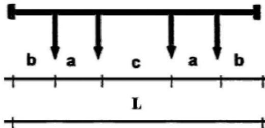
Figura 1: Schema geometrico di un carro
