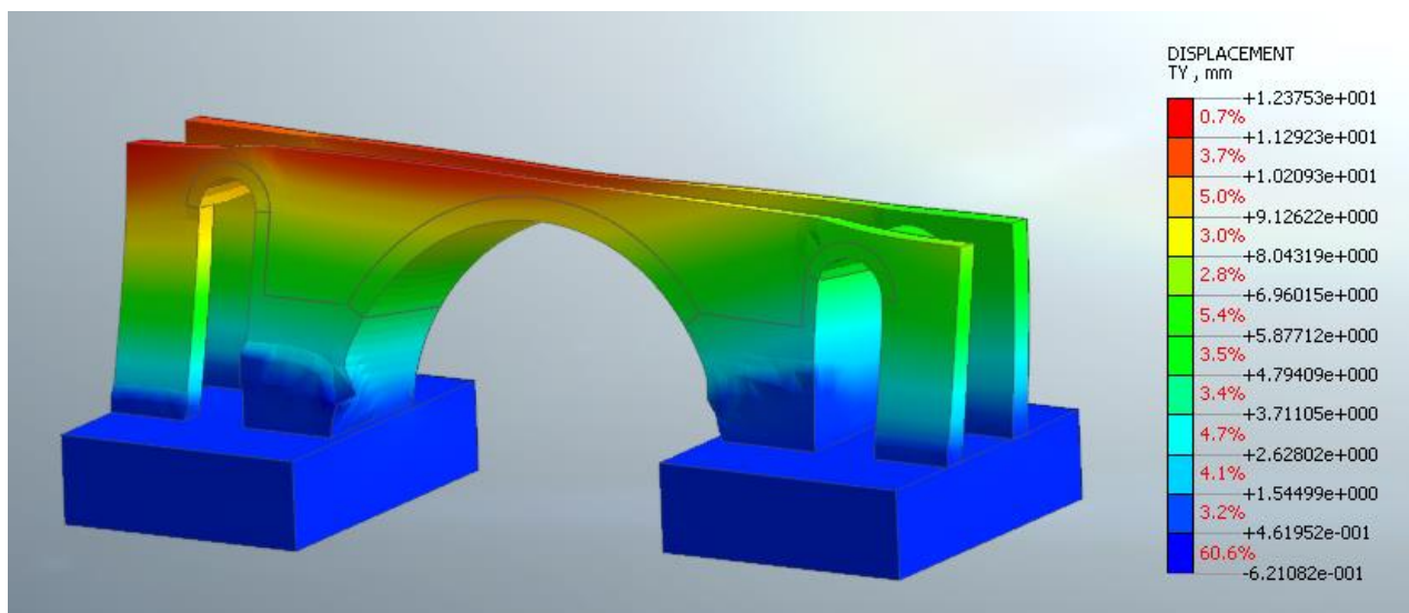
Figura 36: Deformata allo step di collasso
