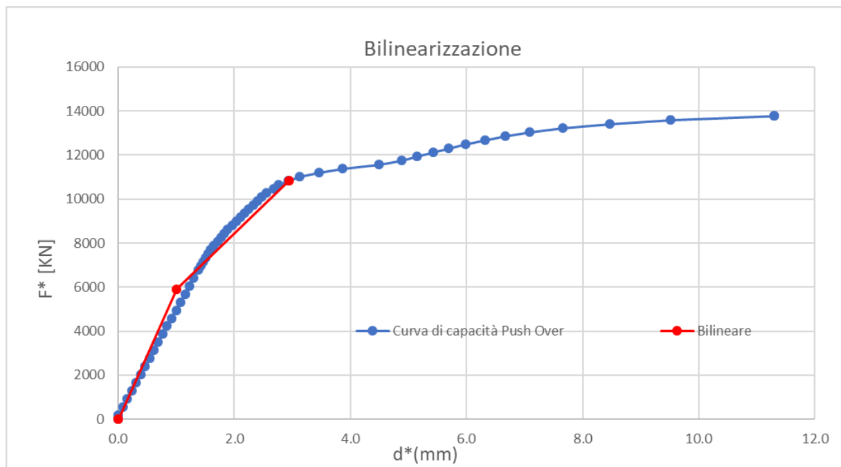
Figura 27: Bilinearizzazione curva di capacità 1GDL.
