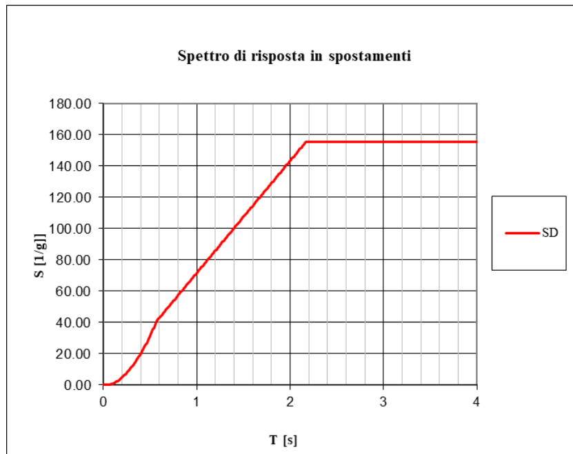
Figura 10: Spettro spostamenti orizzontali
