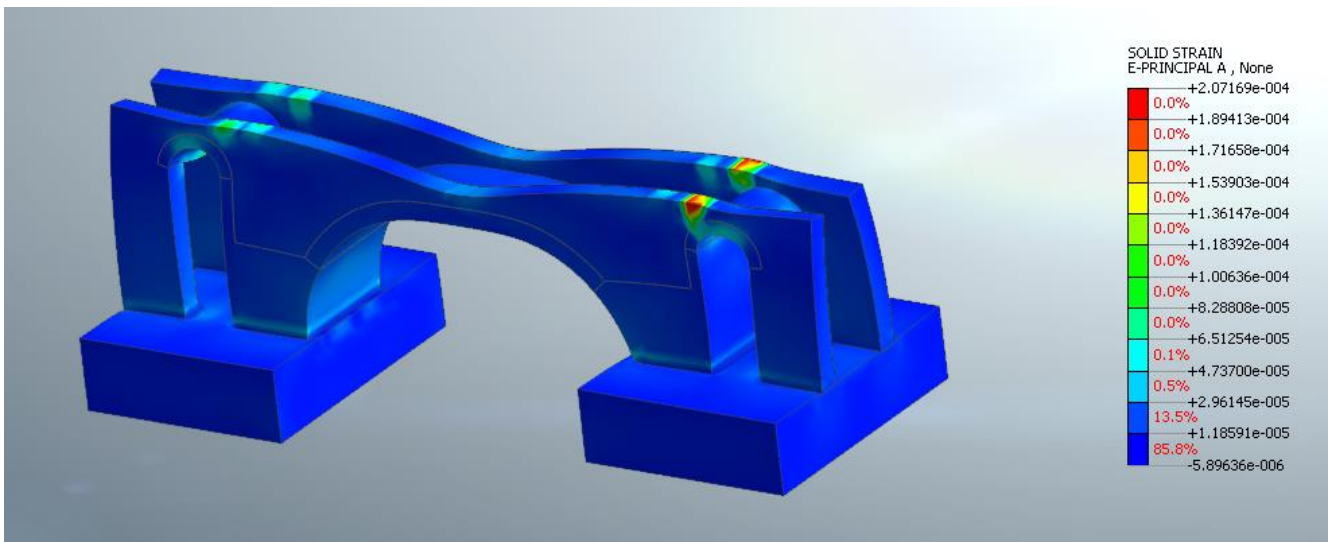
Figura 14: deformazioni massime di trazione (moltiplicatore del carico pari a 1)
