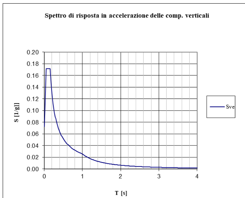
Figura 11: Spettro accelerazioni verticali
