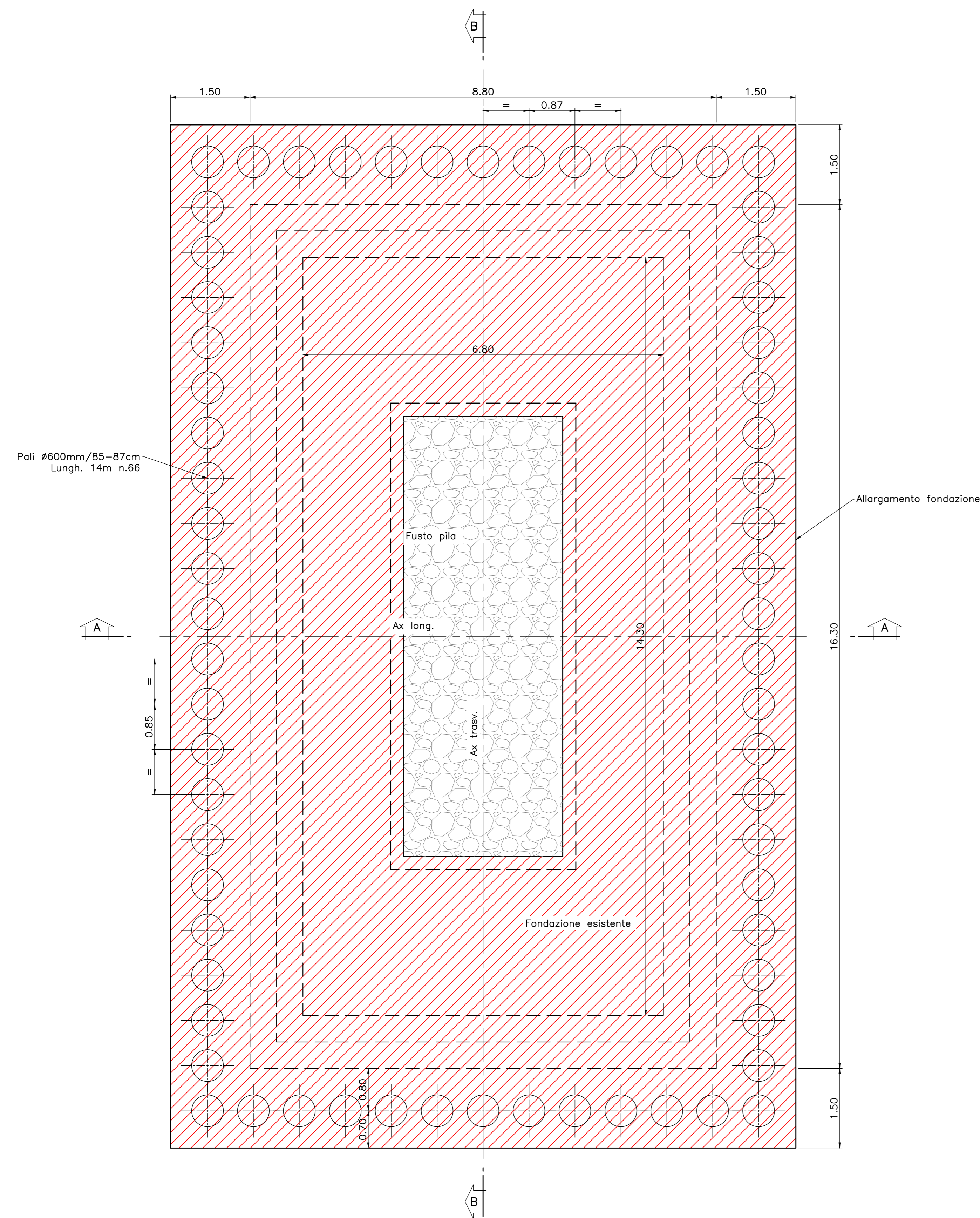
Pianta fondazione Scala 1:50
