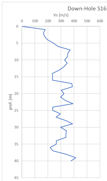
Figura 13: risultati prova Down-Hole
