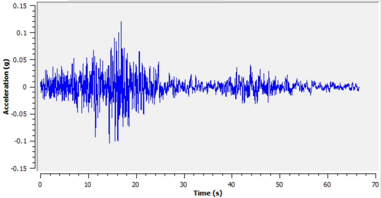
Figura 5: Accelerogramma 000292xa
