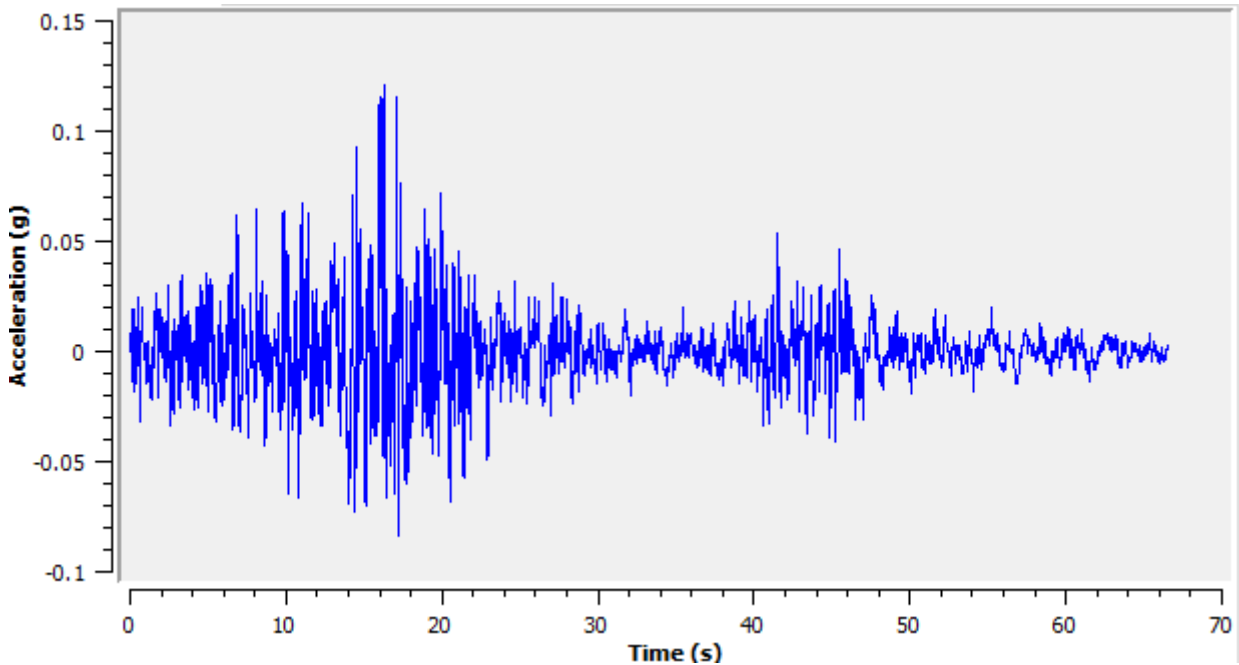
Figura 6: Accelerogramma 000292ya
