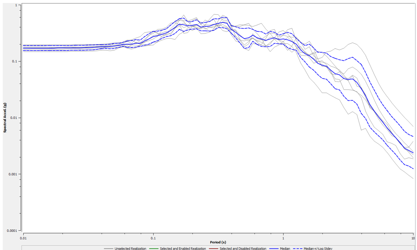
Figura 16: spettro in superficie (Output STRATA)
