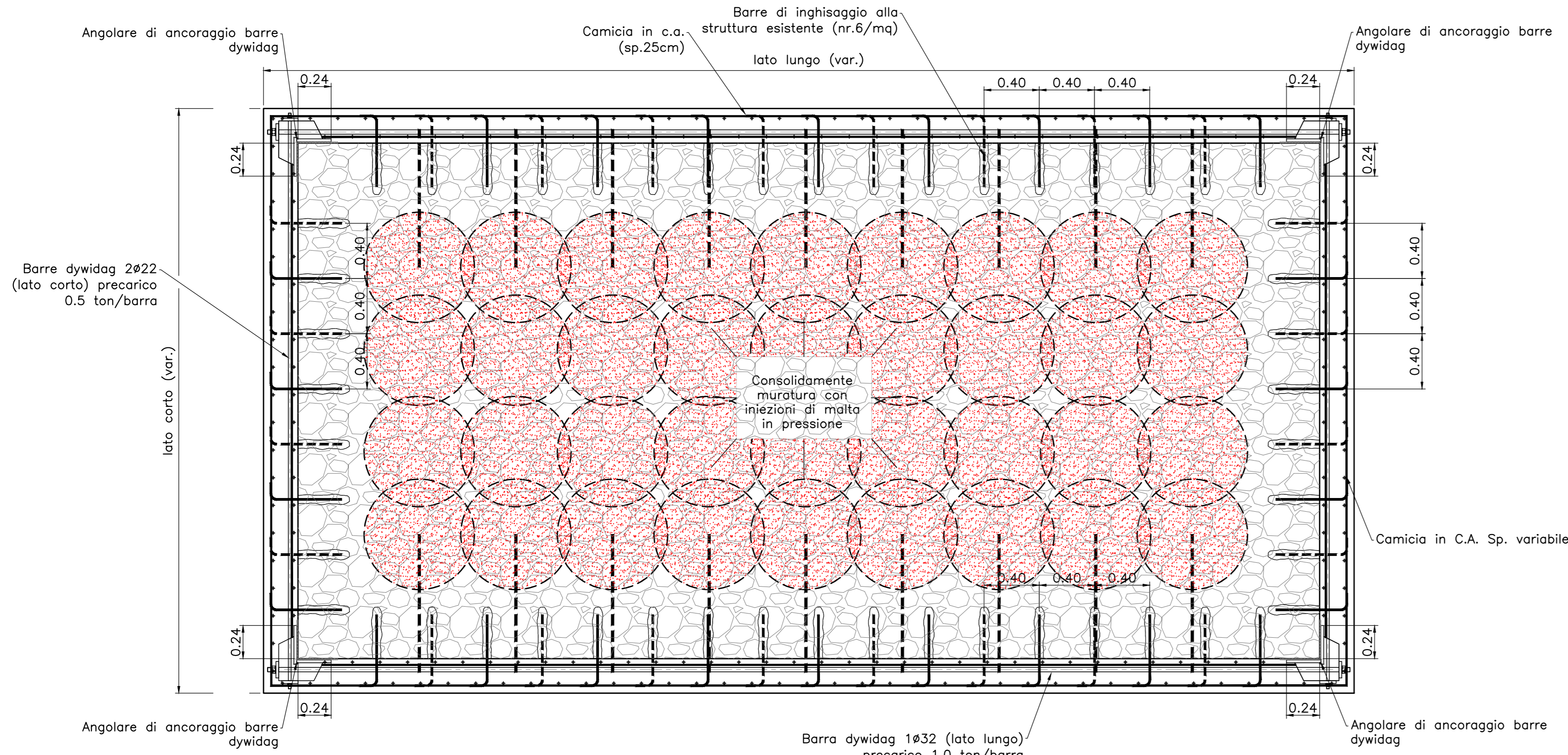
Sezione C-C Scala 1:25
