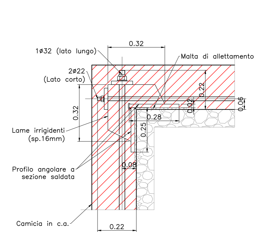
Dettaglio ancoraggio barre dywidag Scala 1:10
