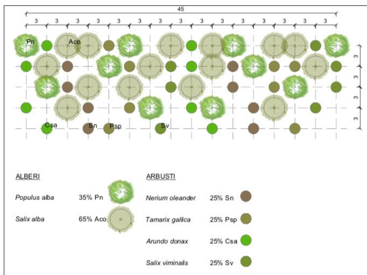
Figura 4-1. Fascia mesoigrofila di compensazione ambientale – Sesto di impianto e quantitativo specie
