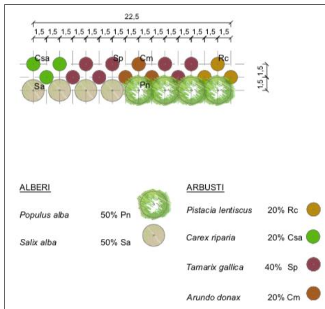
Figura 4-2. Fascia ripariale di mitigazione sistemazioni spondali – Sesto di impianto e quantitativo specie
