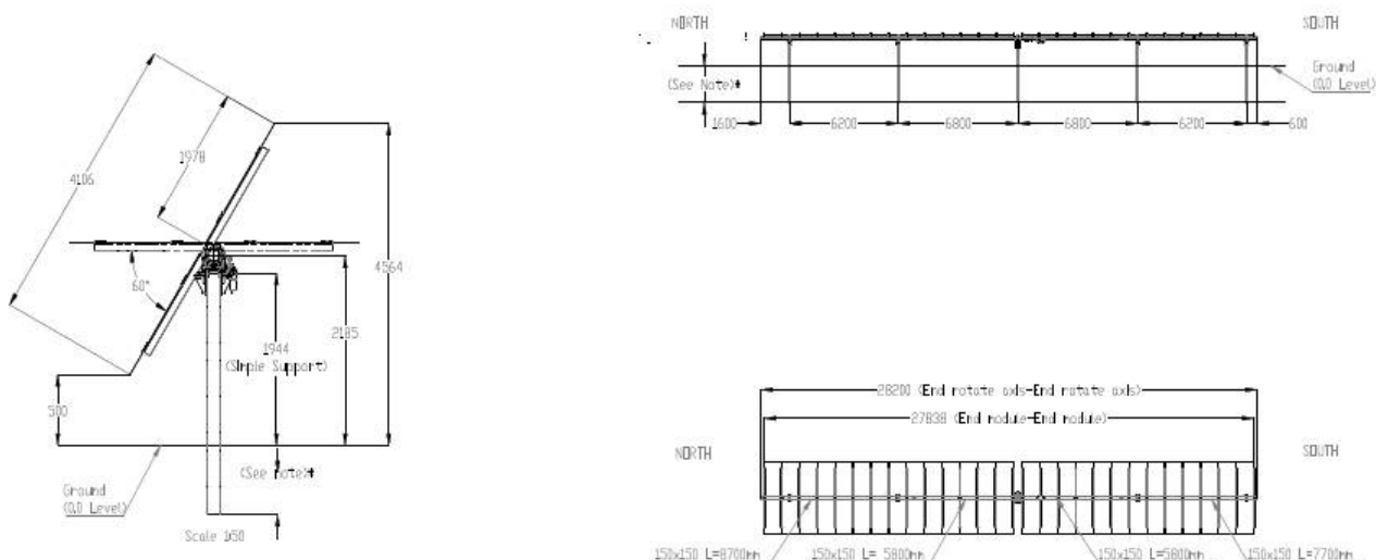
Figura 4 - Strutture Tracker a pali infissi
