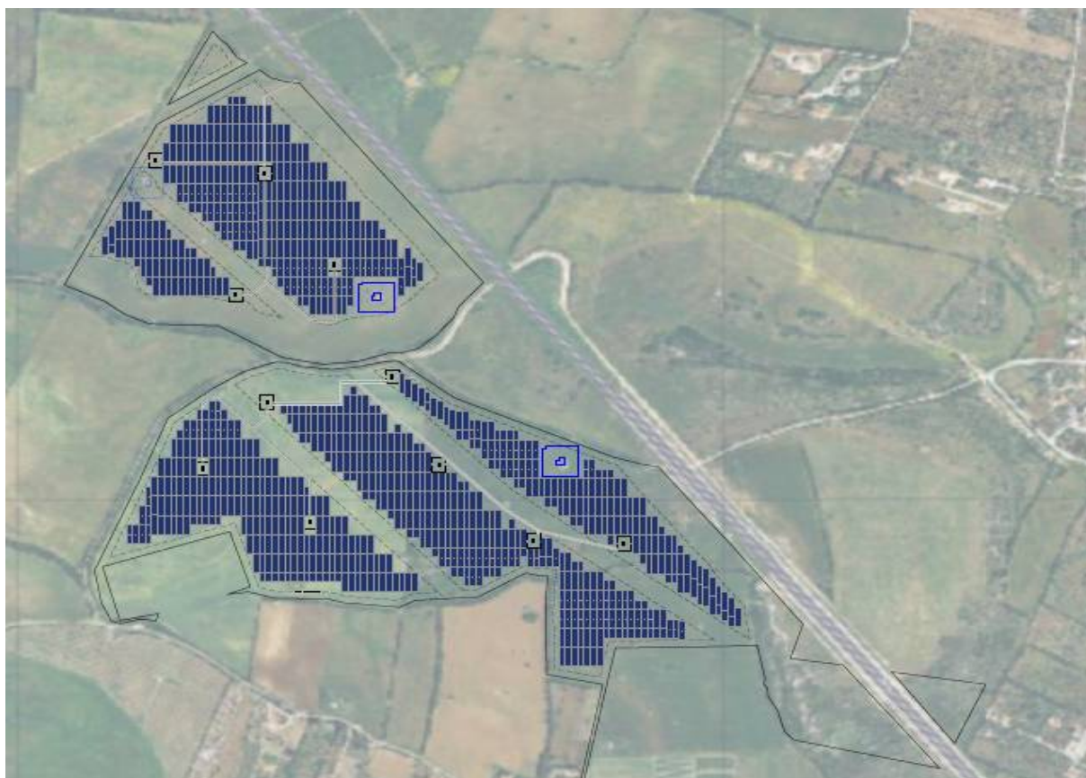
Figura 2 - Areale intervento con impianto fotovoltaico Truncu Reale 3
