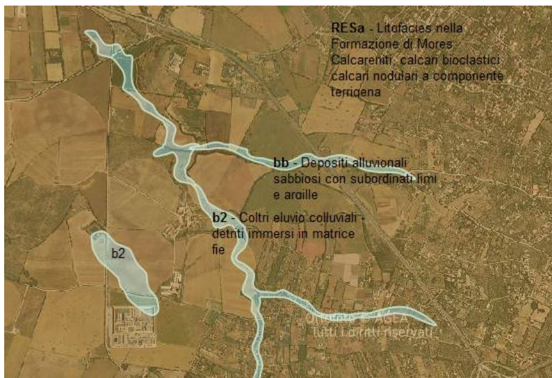
Figura 9 – Inquadramento geologico sc 1:25.000 (fonte Sardegna geoportale)
