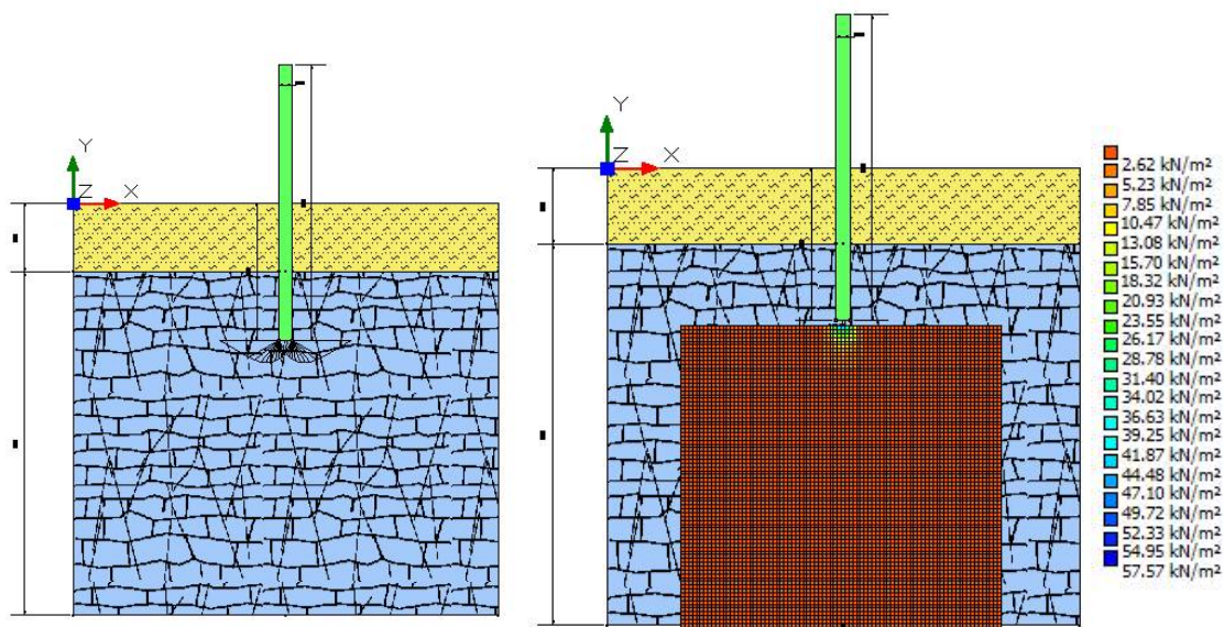
Figura 13 – Cuneo di intrusione / Bulbo delle pressioni
