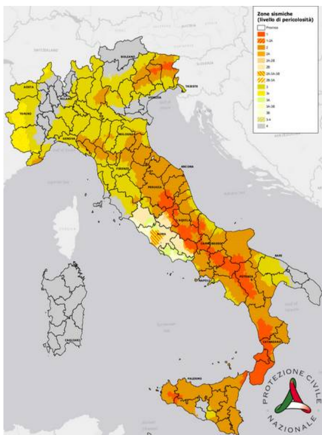
Figura 12 - Livello di pericolosità sismica dei Comuni italiani (2020)
