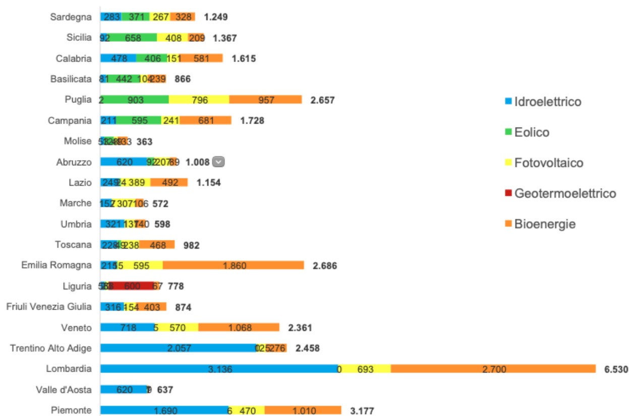
9: Stima delle Unità del Lavoro (ULA) permanenti nel settore della produzione di energia elettrica da FER nel 2020 per regione – fonte GSE.
