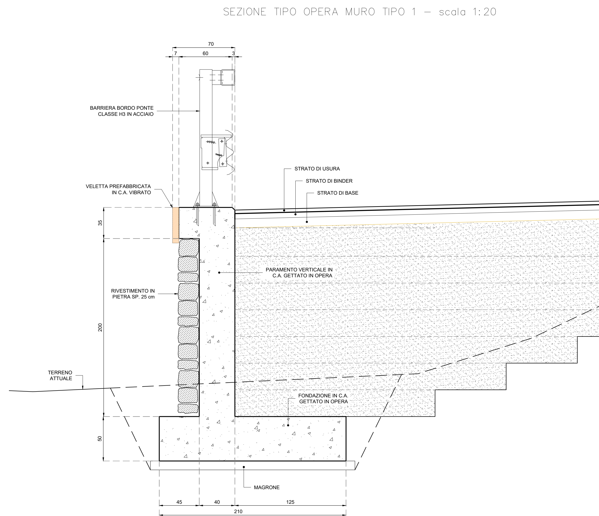
SEZIONE TIPO OPERA MURO TIPO 1 - scala 1:20
