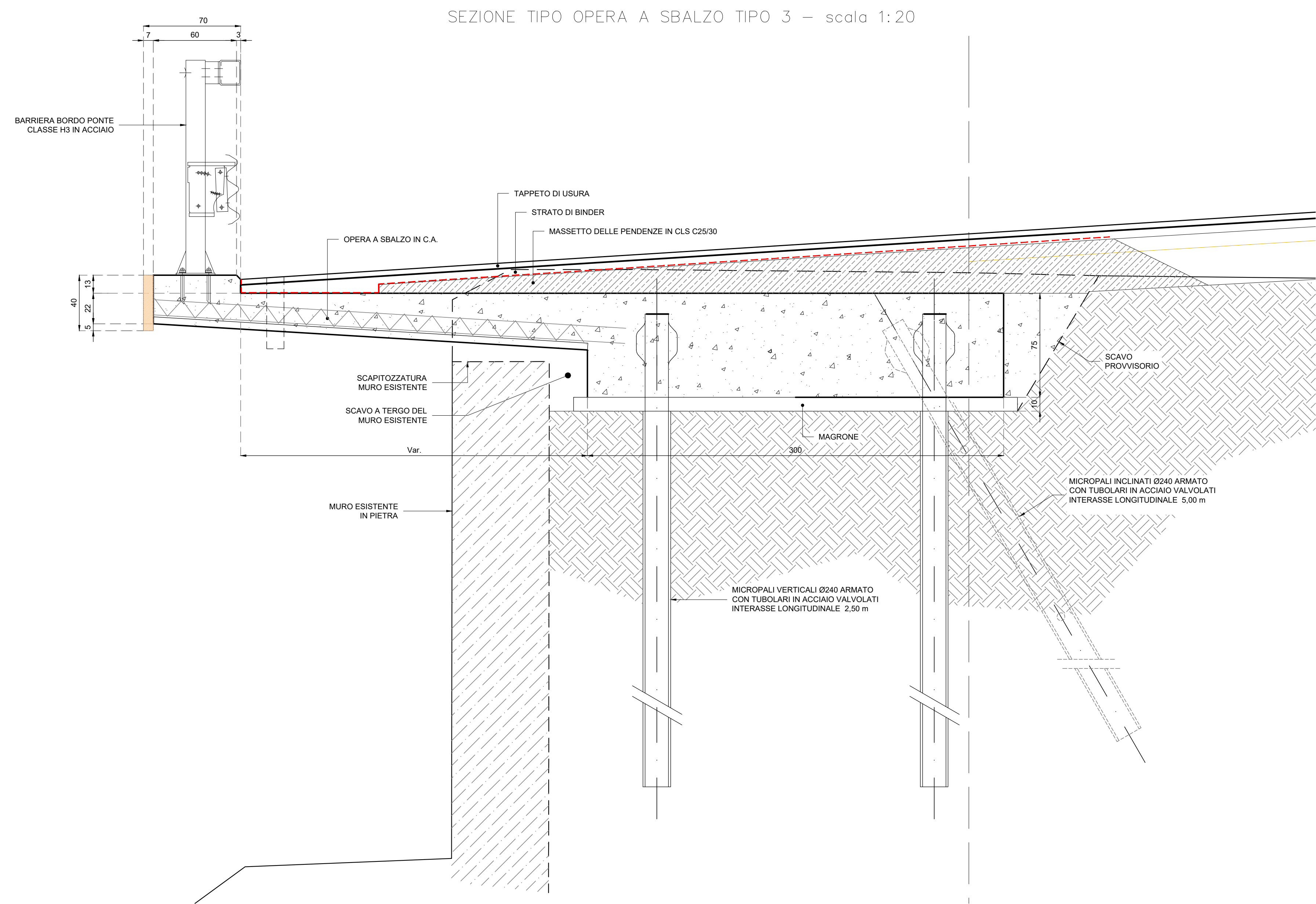
SEZIONE TIPO OPERA A SBALZO TIPO 3 - scala 1:20
