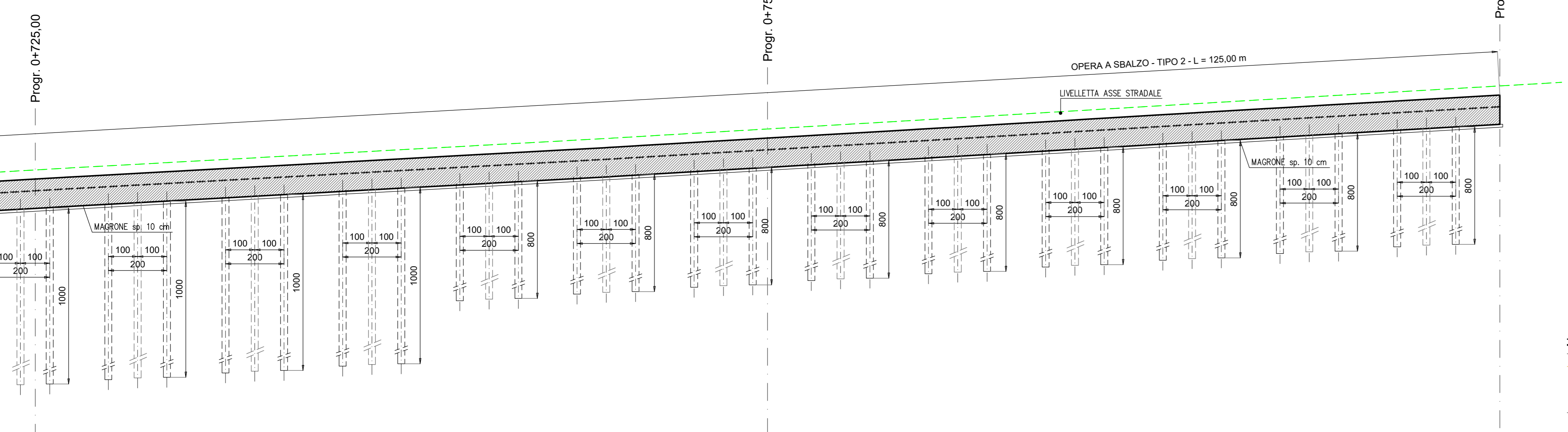
PROSPETTO - Parte 8 di 8 - scala 1:100
