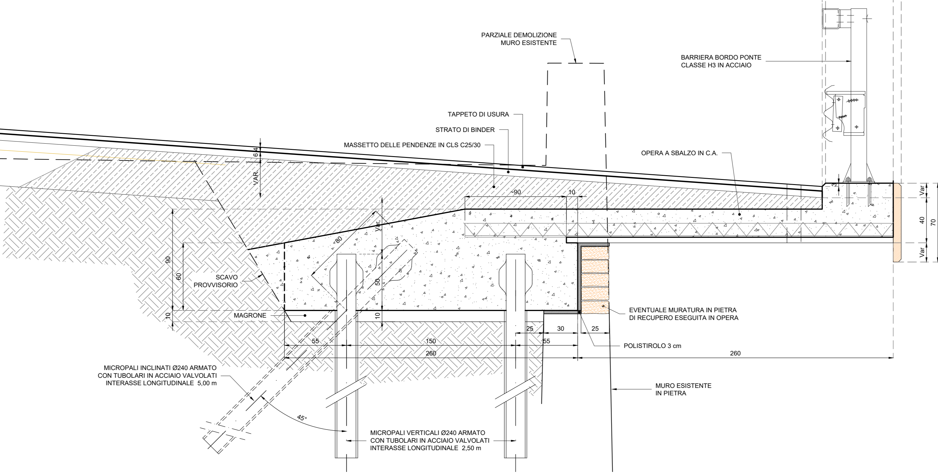
SEZIONE TIPO OPERA A SBALZO "TIPO 1" - scala 1:20
