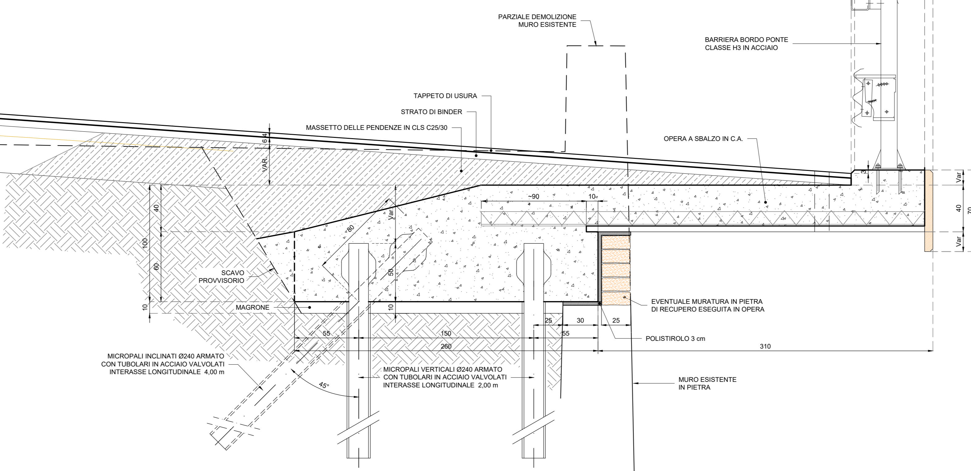
SEZIONE TIPO OPERA A SBALZO "TIPO 2" - scala 1:20
