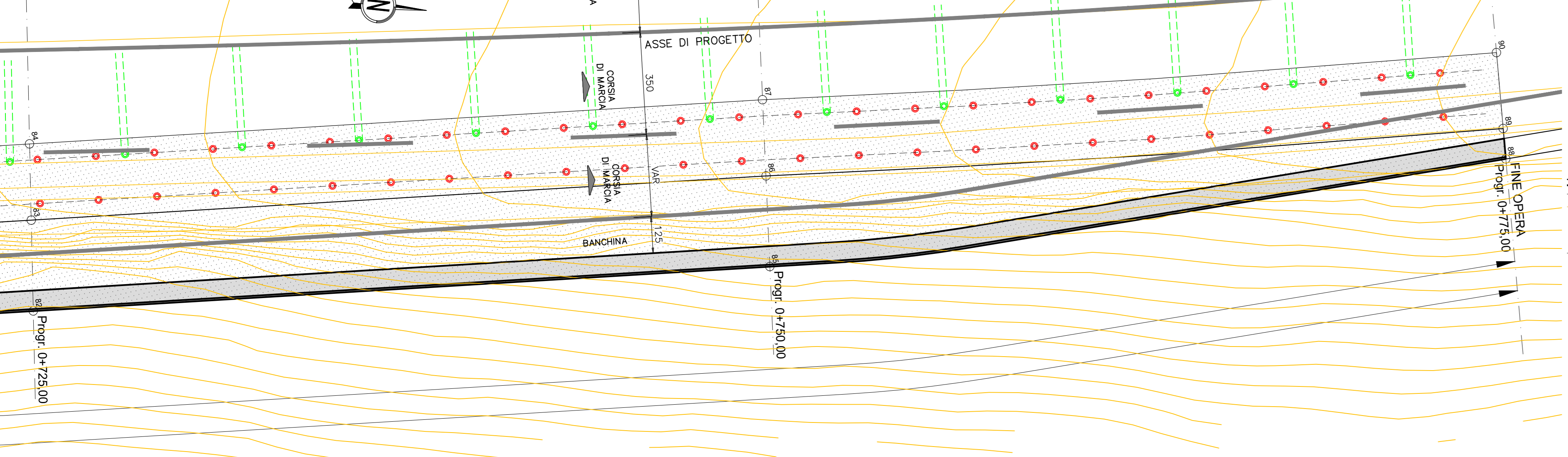
PROSPETTO - Parte 8 di 8 - scala 1:100
