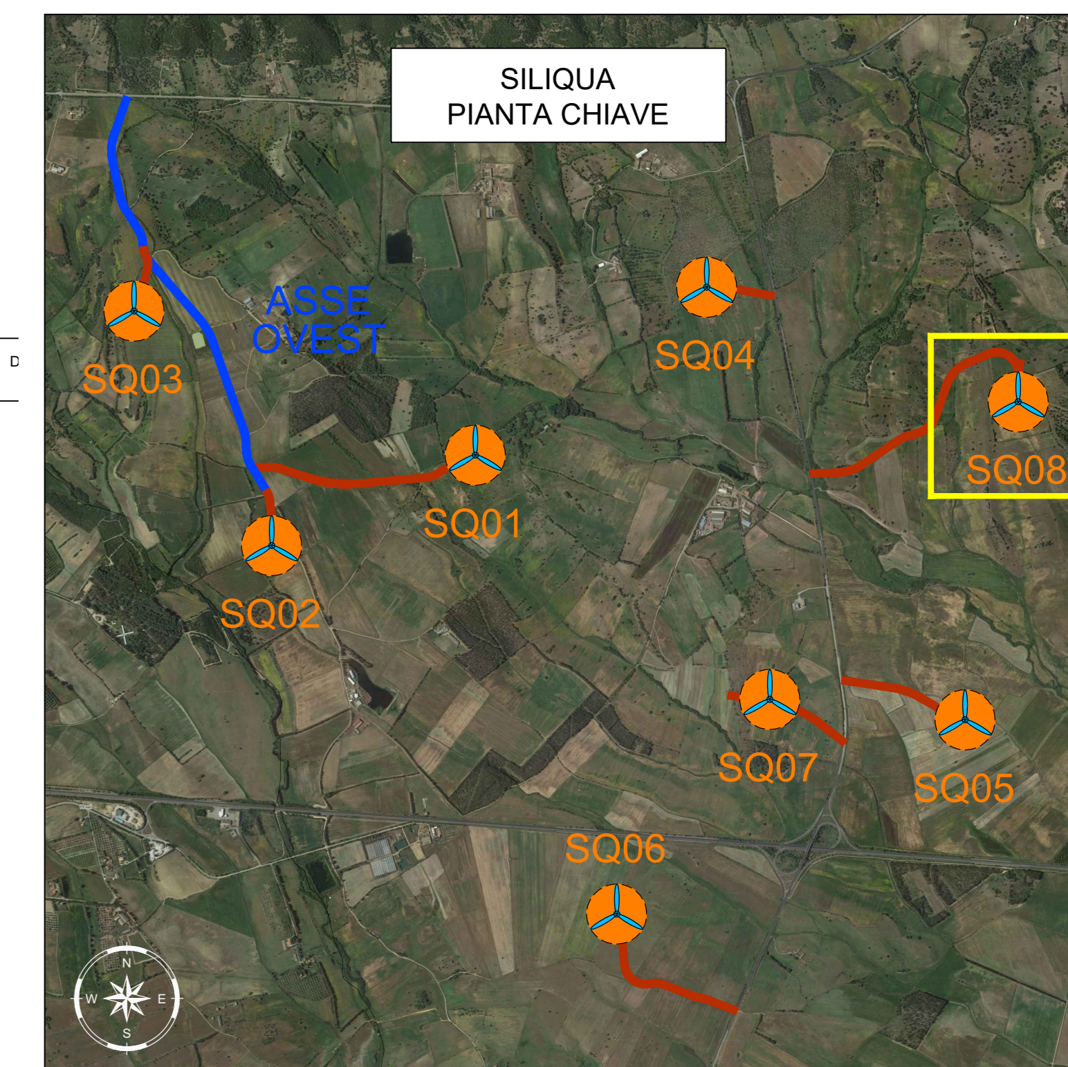
LEGENDA PIANTA CHIAVE PIAZZOLA CON ROTORE EOLICO PISTA DI ACCESSO ALLA PIAZZOLA VIABILITA' ESISTENTE DA ADEGUIARE
