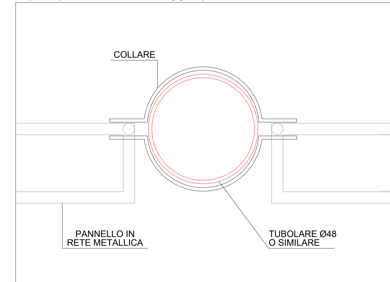
Tipico particolare montaggio pannelli - Scala 1:2
