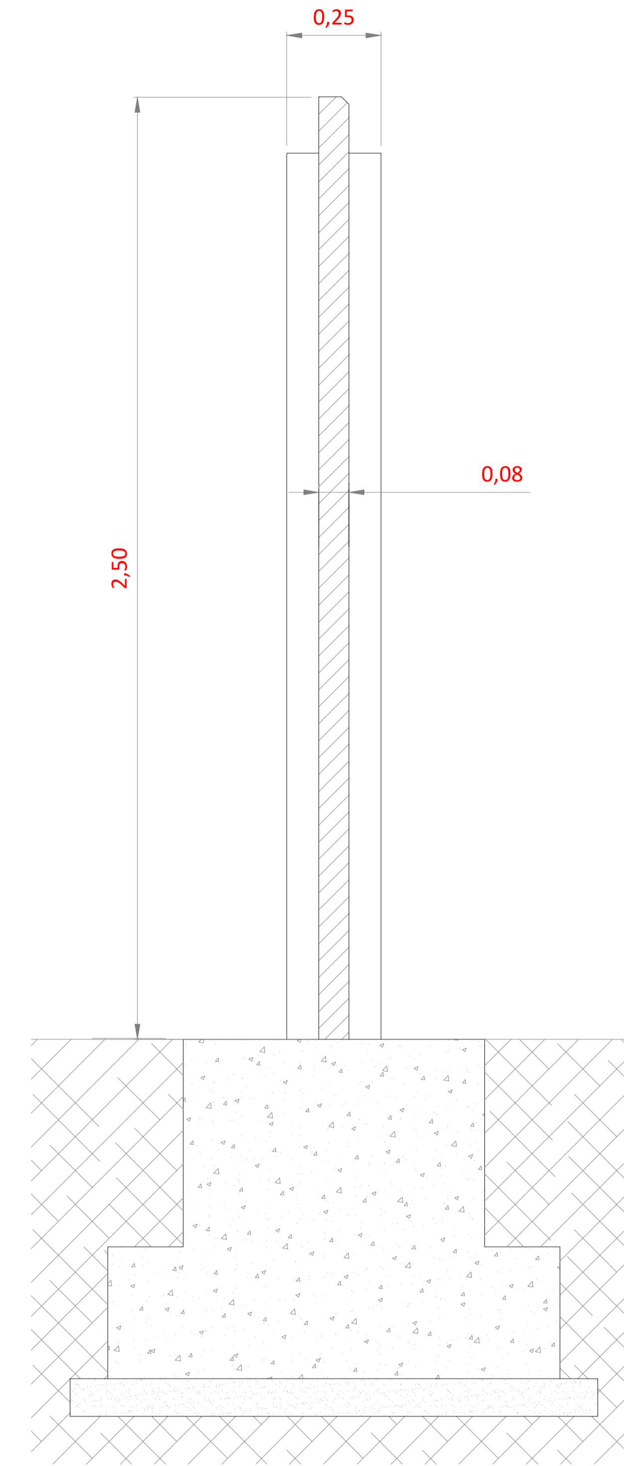
SEZIONE A-A
