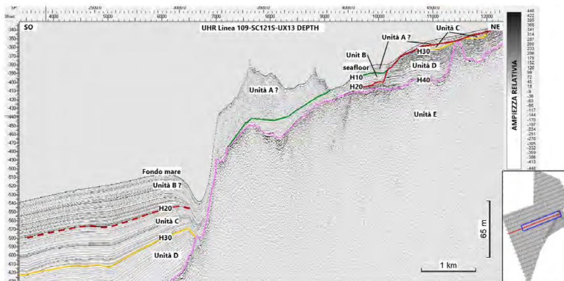
Figura 2.9: Esempio di dato UHR (Linea 109-SC121S-UX13 DEPTH)
