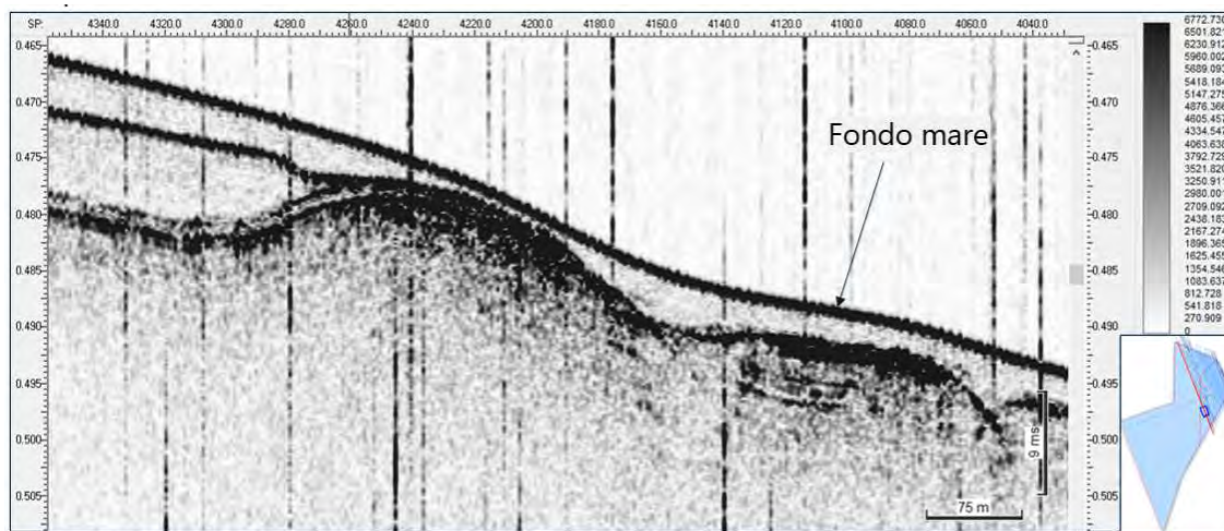
Figura 2.7: Esempio di SBP sullo scafo (Linea SC121S-U072_HMC)
