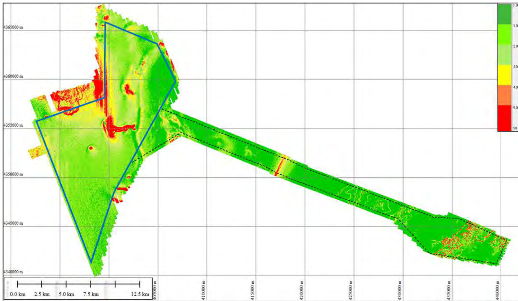
Figura 2.2: Gradiente del fondale marino dell'area del rilievo (linea blue: Sito Principale)
