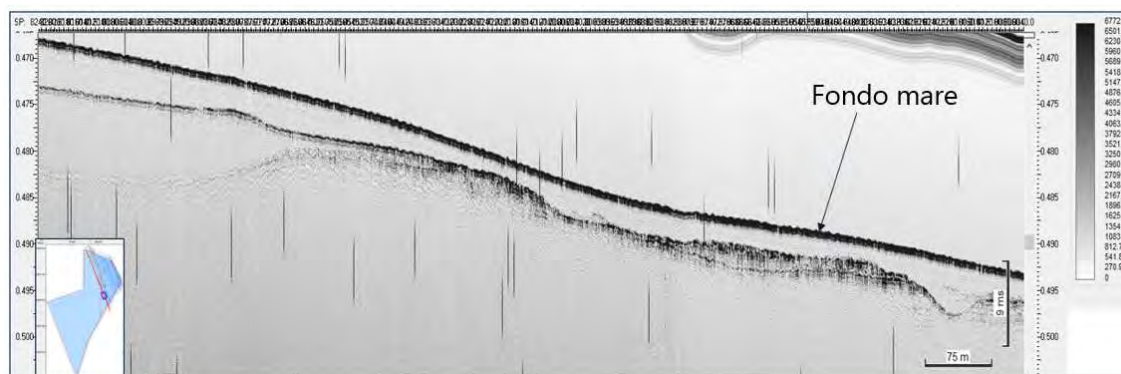
Figura 2.8: Esempio di SBP a traino (Linea SC121S-U072_FC)
