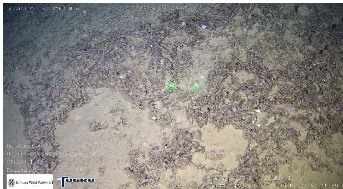
Figura 2.11: Possibile formazione rocciosa biogenica/vulcanica [SC21S_03_T01]
