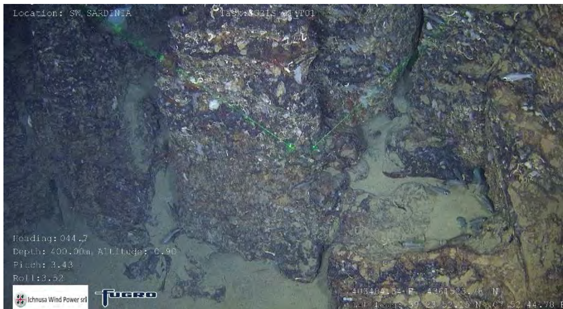
Figura 2.12: Affioramento roccioso[SC21S_01_T01]
