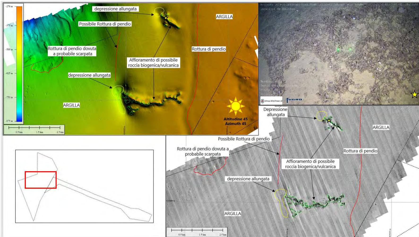
Figura 2.3: Esempi di MBES, SSS e immagine ROV del settore centrale del sito principale
