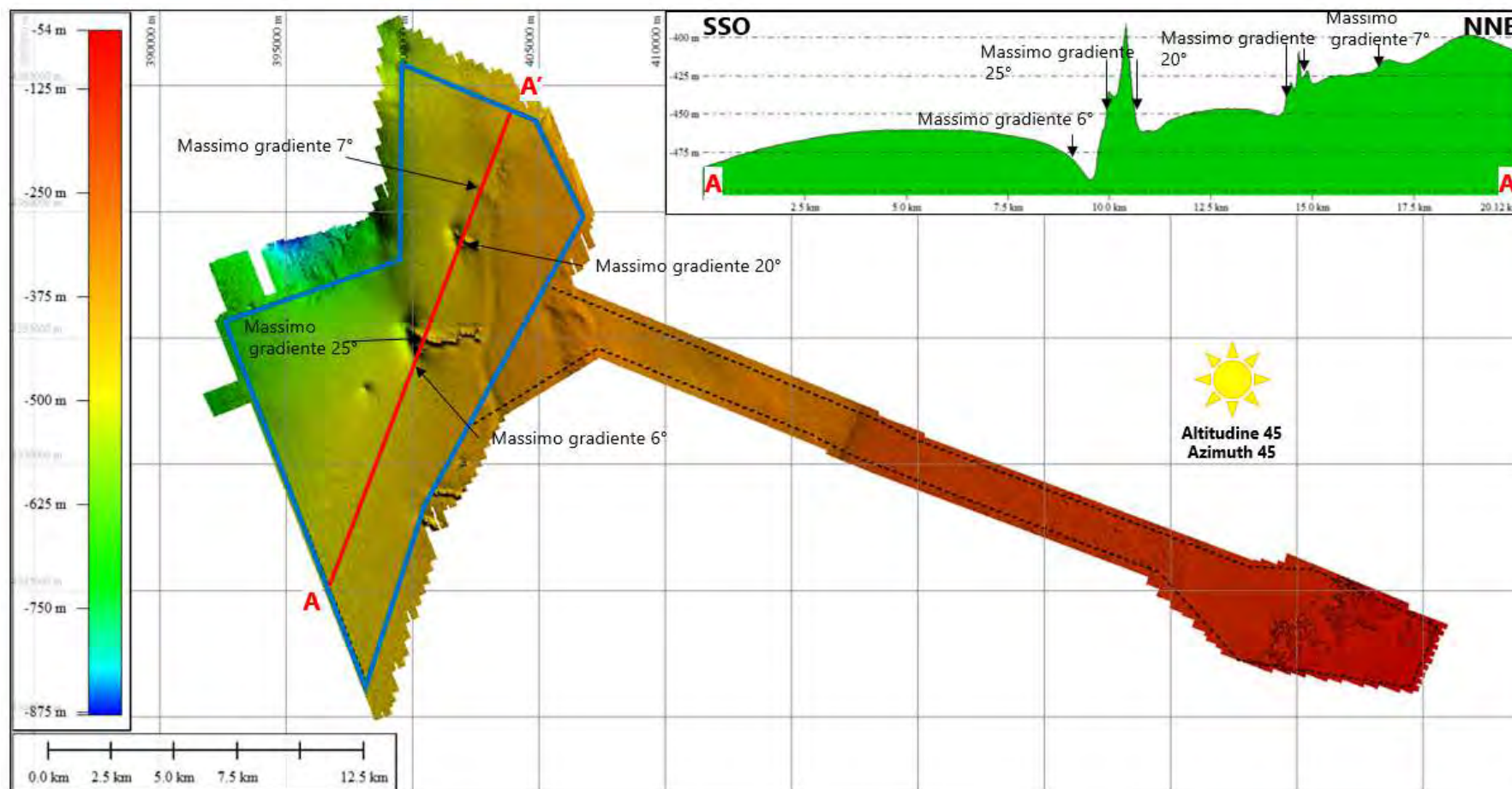
Figura 2.1: DTM (MBES) finale dell'area del rilievo e profili bati-morfologici lungo il sito principale (linea rossa)
