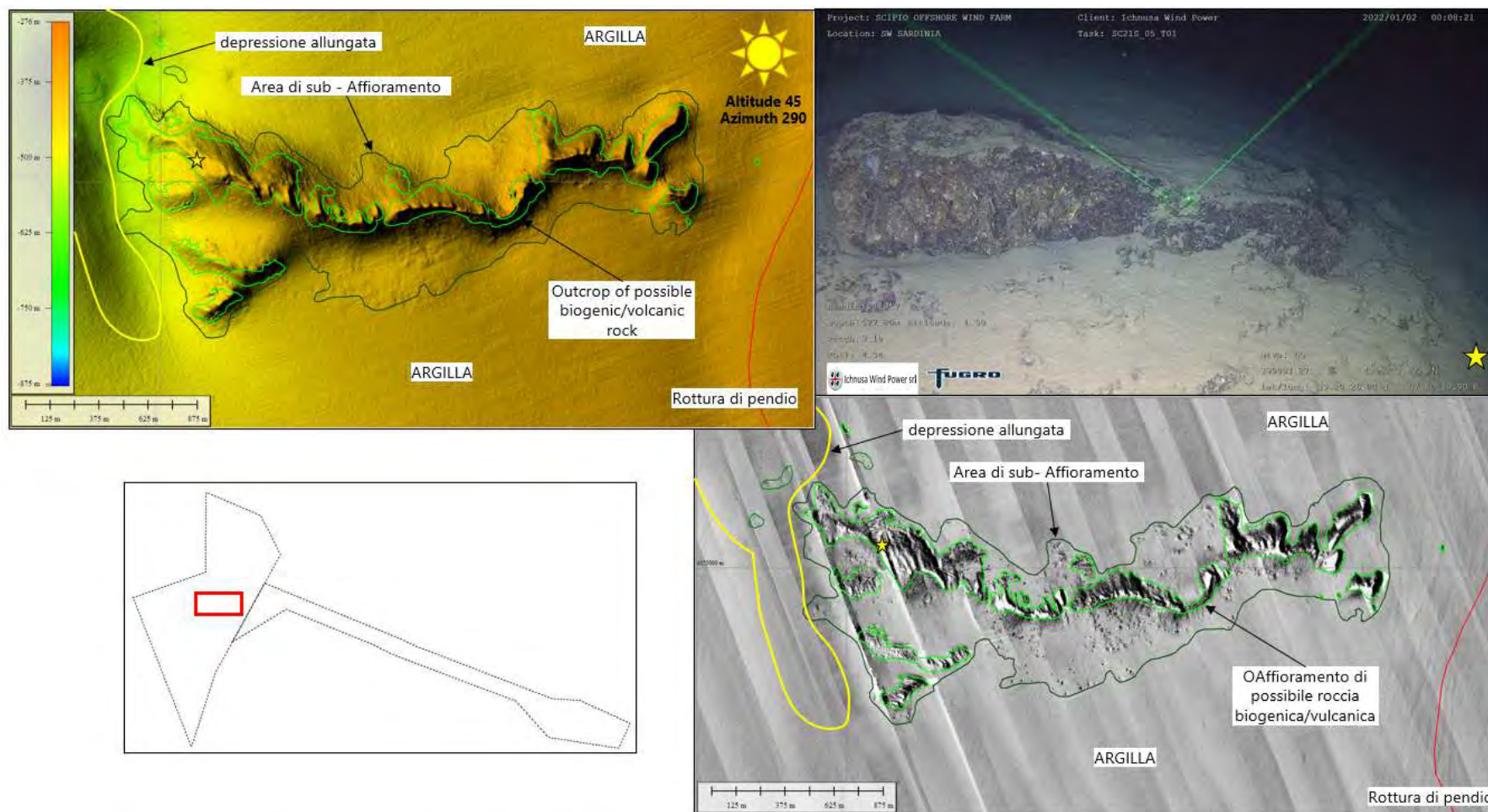
Figura 2.4: Esempi di MBES, SSS e immagine ROV dell' affioramento di possibile roccia biogenica/vulcanica con area circostante di sub-affioramento nel settore centrale
