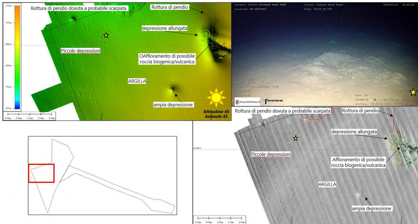
Figura 2.5: Esempi di MBES, SSS e immagini ROV dell' area delle depressioni presenti nel settore occidentale e centrale del sito principale
