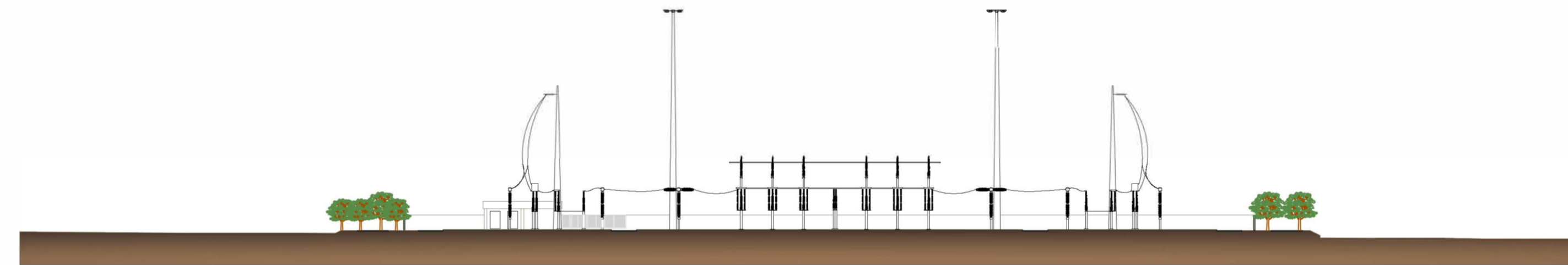
Sezione B-B
