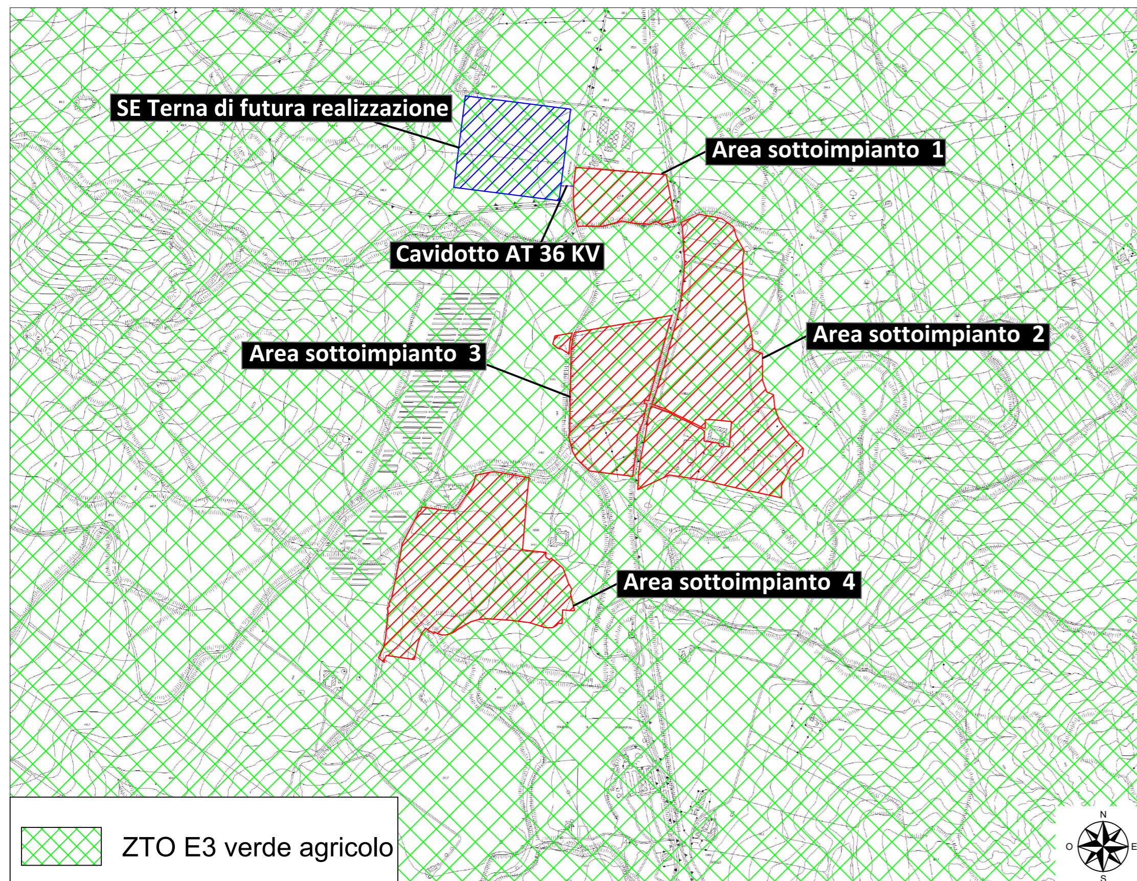
Stralcio Zonizzazione del comune di Villalba (CL). Scala 1:10.000
