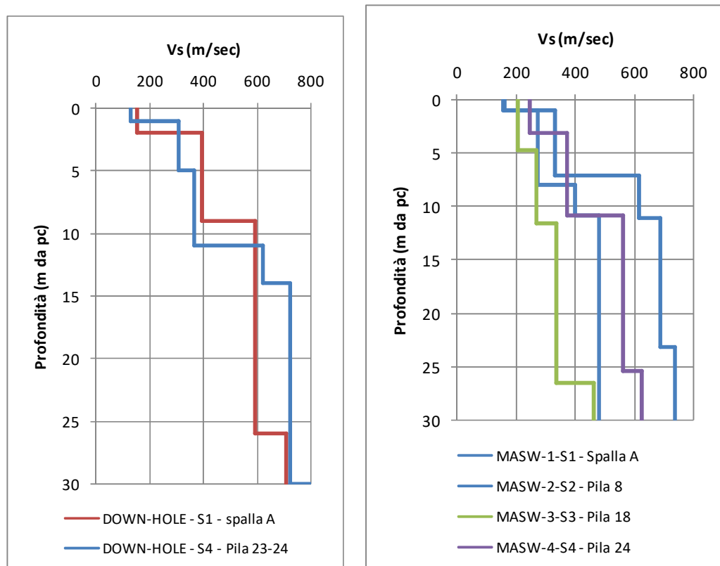
Andamento dei valori di Vs (prove DOWN-HOLE e MASW)
