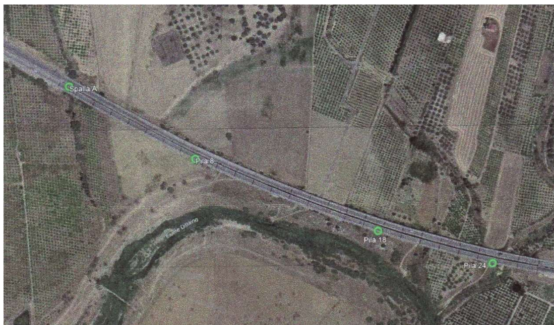
Ubicazione dei sondaggi geognostici
