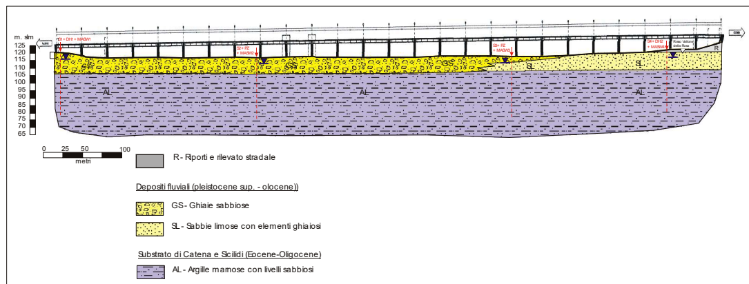
Sezione stratigrafica
