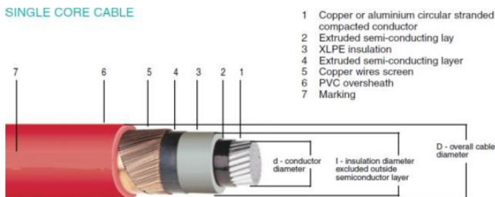
Figura 4-1: Caratteristiche cavi MT
