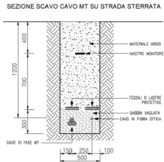
Figura 4-2: Sezione tipica di posa della linea in cavo su strade sterrate
