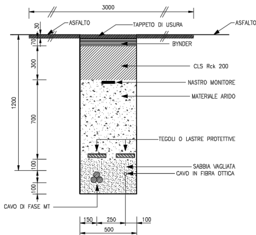
SEZIONE SCAVO CAVO MT SU STRADA ASFALTATA
