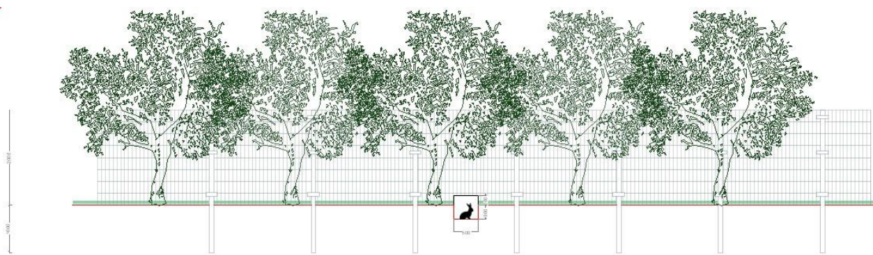
Figura 9. Particolare dei sottopassaggi faunistici
