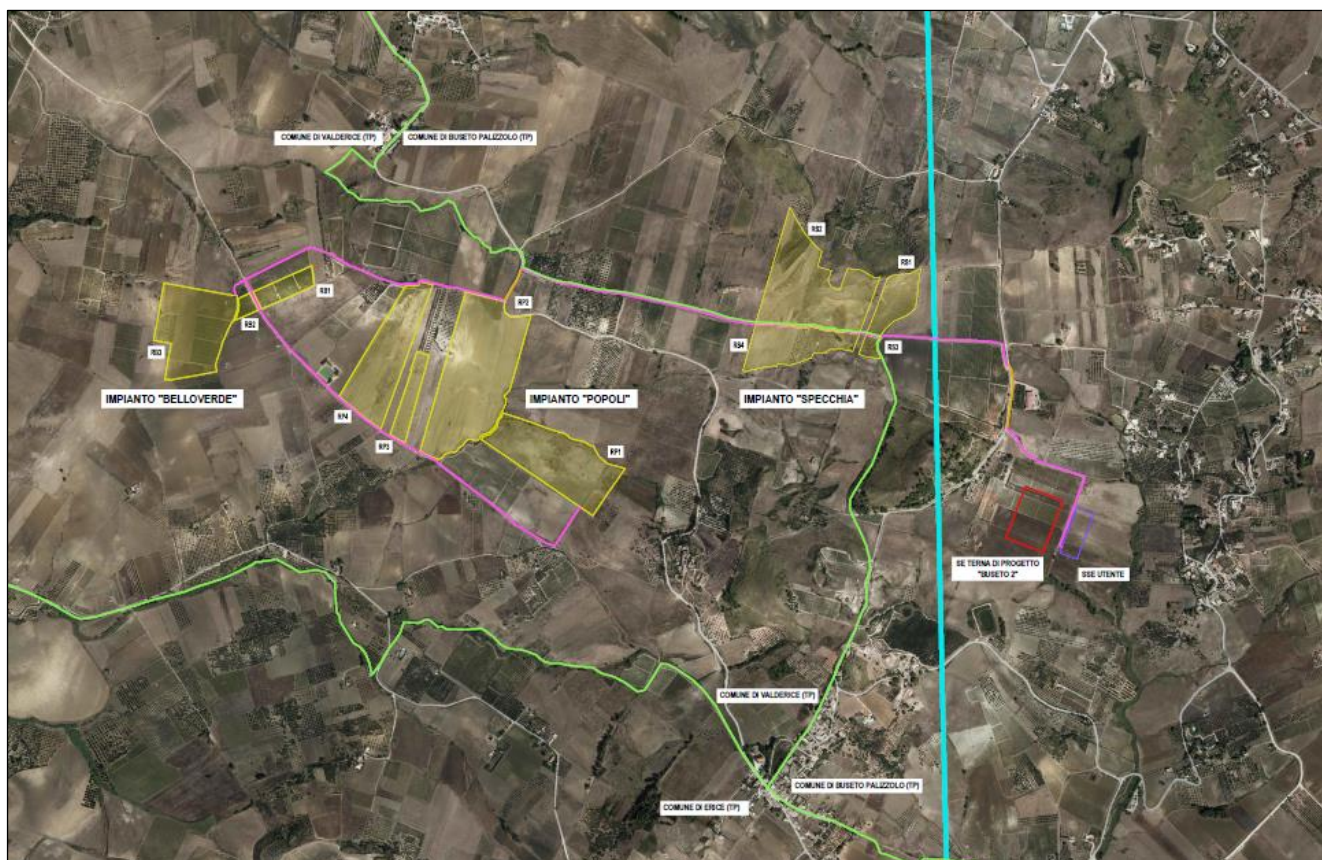
Figura 2. Inquadratura opere in progetto su Ortofoto (Scala 1:10000)
