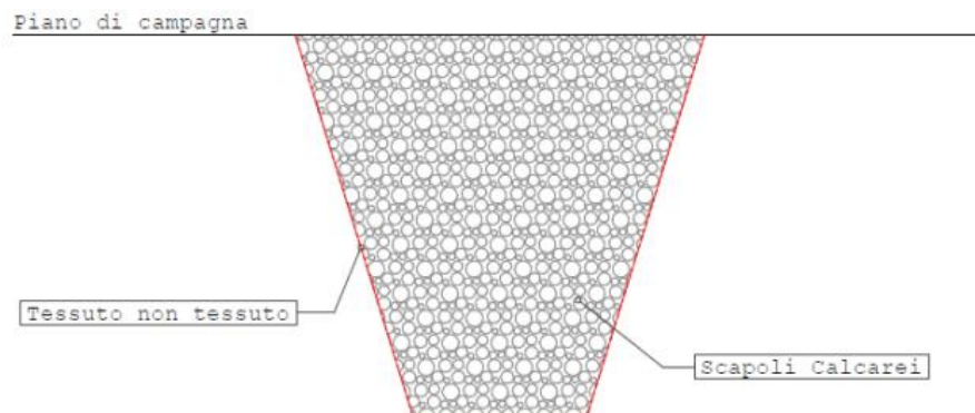
Figura 4.Sez. tipo Trincea drenante
