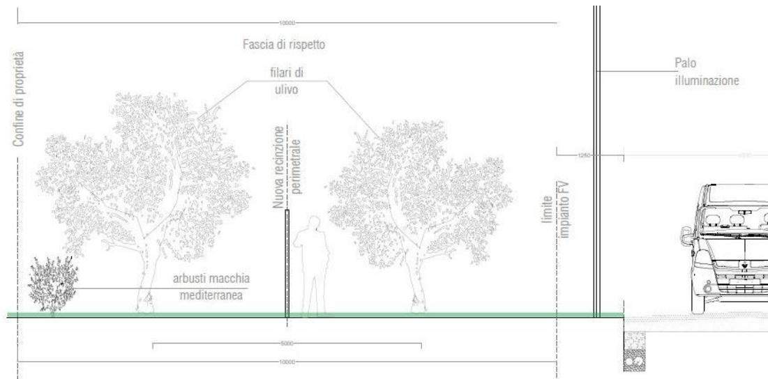
Figura 8. Tipico fascia arborea/arbustiva perimetrale
