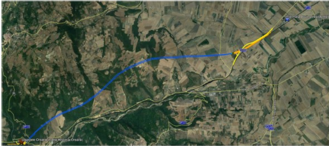
Figura 1-1. Corografia della linea. In blu la tratta in galleria, in arancio la tratta in rilevato ed in giallo le nuove viabilità.
