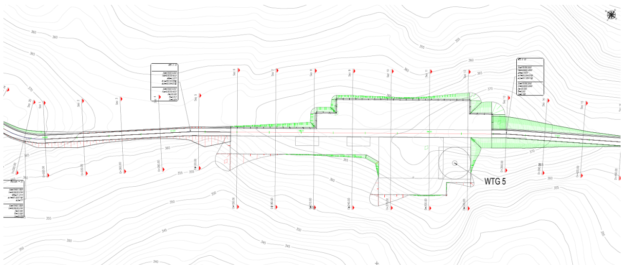
Figura 4: Tracciato planimetrico viabilità di nuova realizzazione. Fonte: elaborato di progetto "GRE.EEC.D.73.IT.W.15235.12.015_Layout strade WTG5-WTG10"
