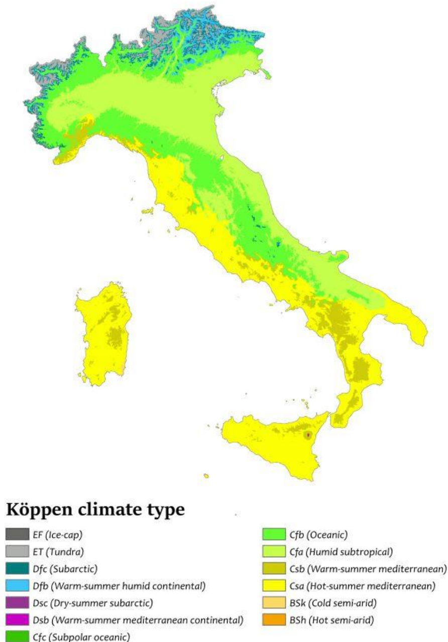
Figura 23 – Classificazione climatica dell'Italia secondo il metodo di Köppen (fonte worldclim.org).
