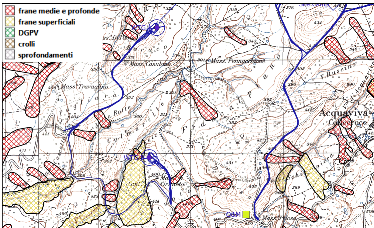
Figura 13: Posizionamento di WTG1 e WTG9 e fenomeni franosi (database dei fenomeni franosi IFFI tratte da
