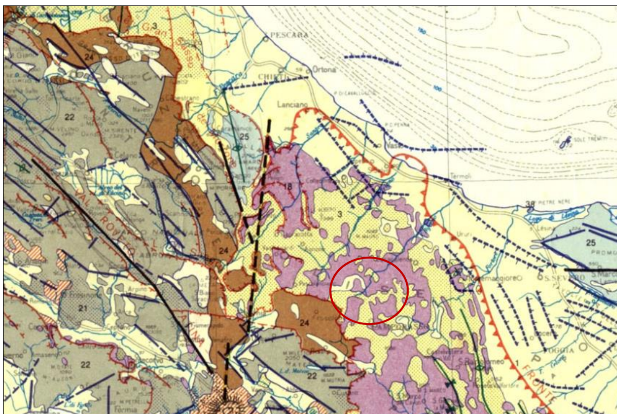
Figura 9: Carta Tettonica d’Italia – Progetto finalizzato GEODINAMICA CNR – sca 1:500.000
