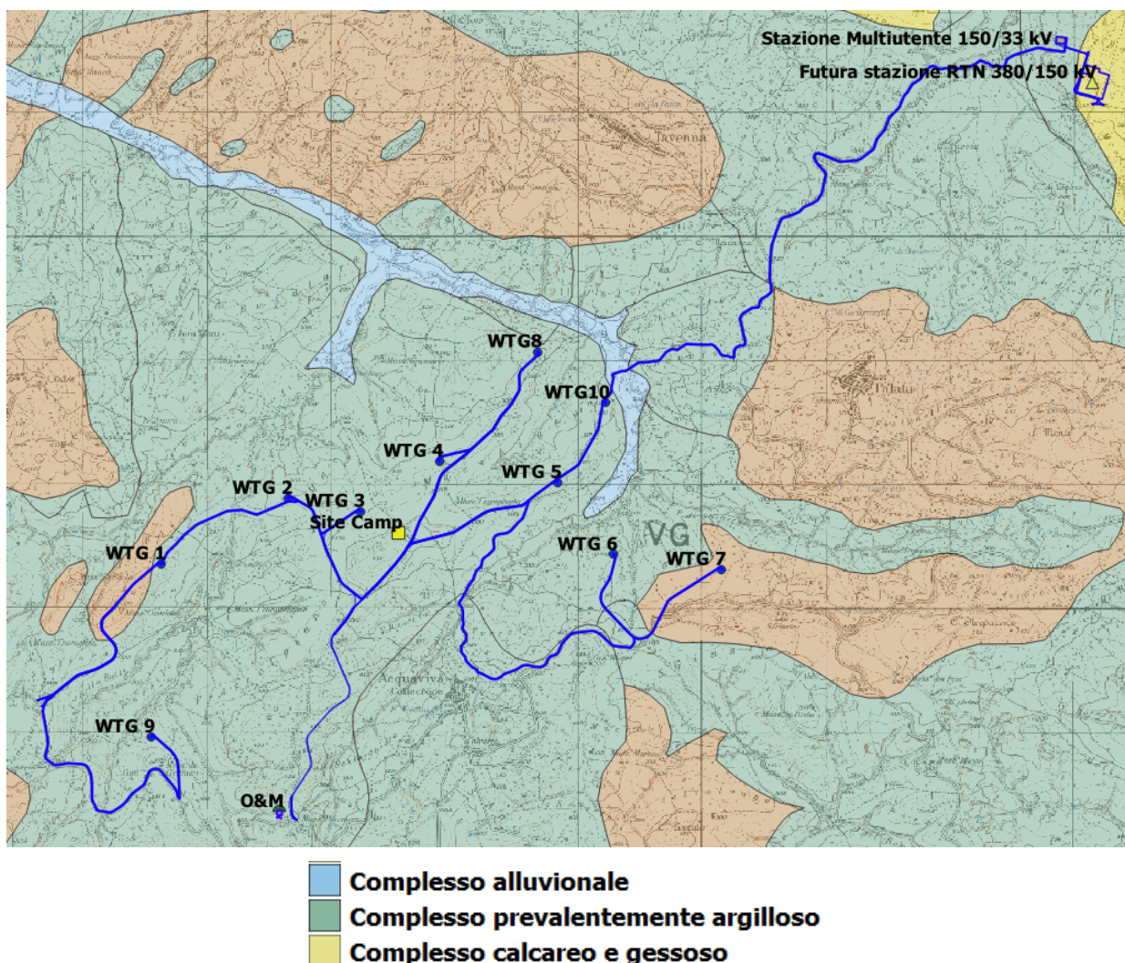
Figura 27: Carta dei complessi idrogeologici, ricostruita sulla base delle litologie riportate nel GeoPortale Nazionale.
