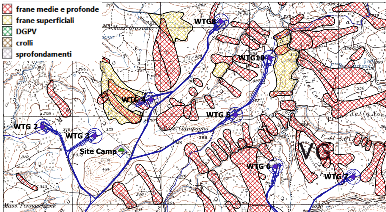
Figura 14: Posizionamento delle WTG (WTG3, WTG4, WTG5, WTG6, WTG7, WTG8, WTG10) e fenomeni franosi (database dei fenomeni franosi IFFI tratte da Geoportale Nazionale).
