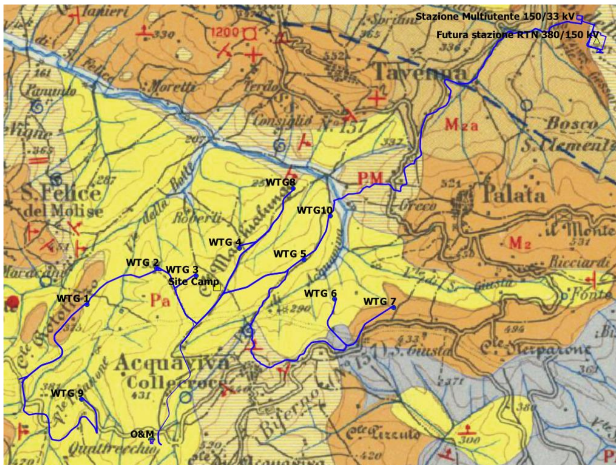
Figura 12: Carta Geologica d'Italia in scala 1:100.000 con ubicazione delle WTG e delle relative opere di connessione
