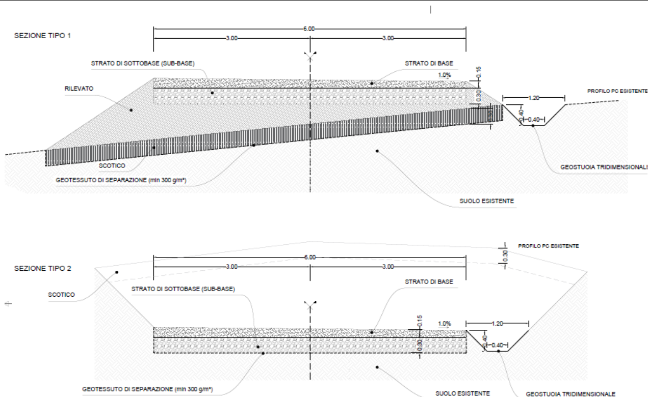
Figura 6: Sezione trasversale viabilità di nuova realizzazione. Fonte: elaborato di progetto “GRE.EEC.D.73.IT.W.15235.12.021_ Sezione stradale tipo e particolari costruttivi”
