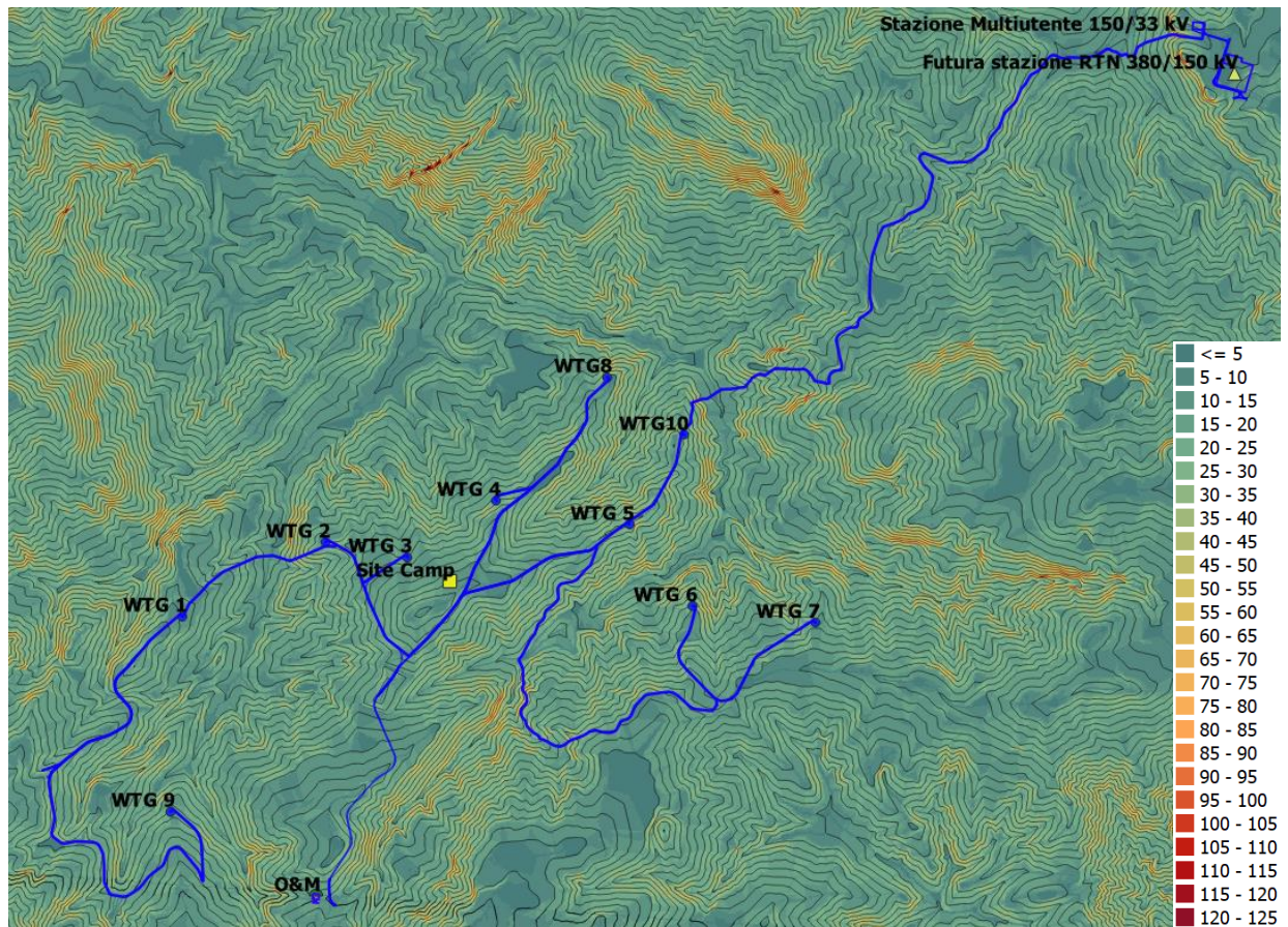
Figura 16: Carta delle pendenze dell'area di diretto interesse e di un suo immediato intorno, tratta dal DTM passo 20 m del Geoportale Nazionale. Pendenze espresse in percentuale.
