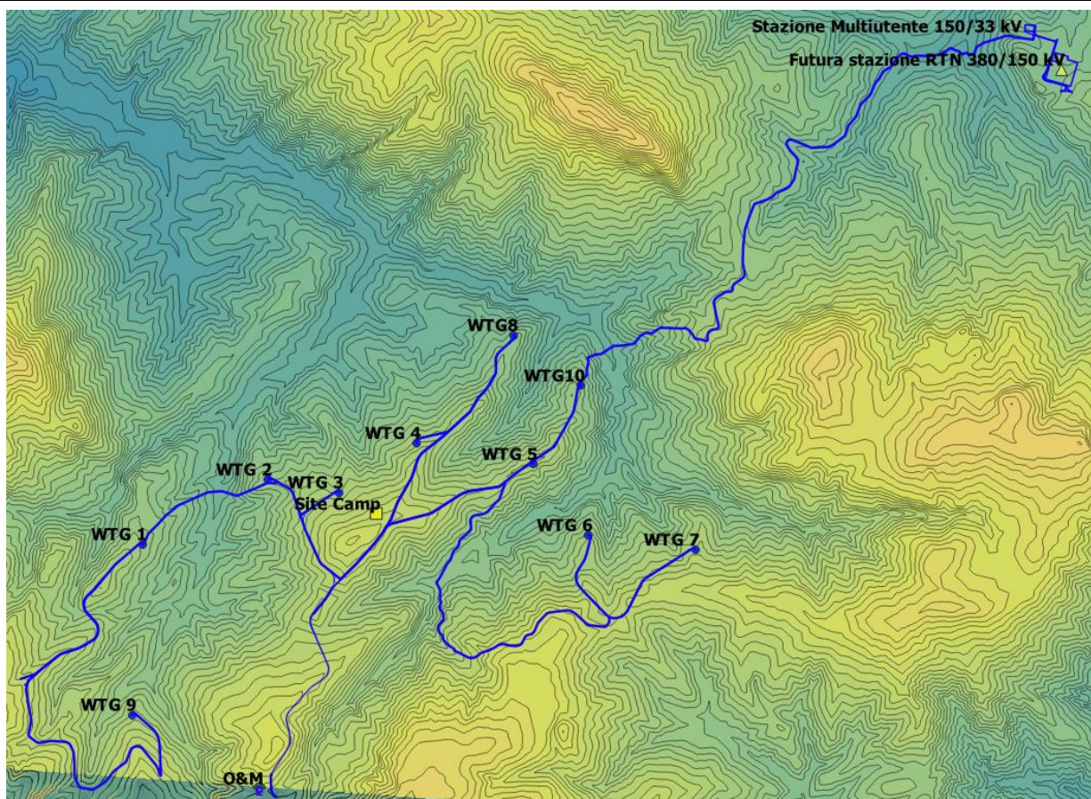
Figura 17: Modello digitale di elevazione del terreno (DTM), con passo 20 m, tratto dal Geoportale Nazionale. Curve di livello con equidistanza 10 m. I toni caldi indicano le quote maggiori.
