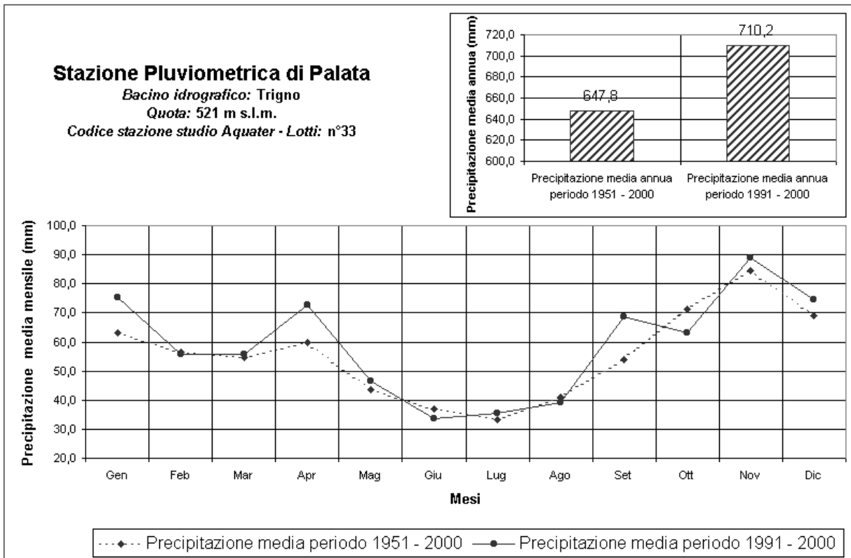
Figura 25: Dati pluviometrici Palata; confronto dati anni 1951-2000 vs anni 1991-2000.
