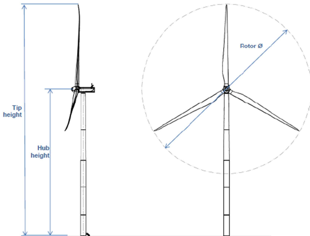
Figura 15. Dimensioni aerogeneratore da 6MW in progetto: Hhub:115m; Rotore:170m; HTip 200m.
