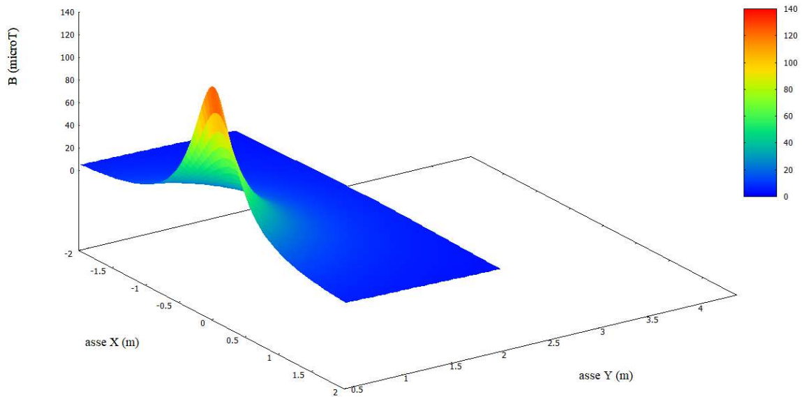
Figura 3. Andamento 3D induzione elettromagnetica per una terna AT interrata 1.6m di profondità
