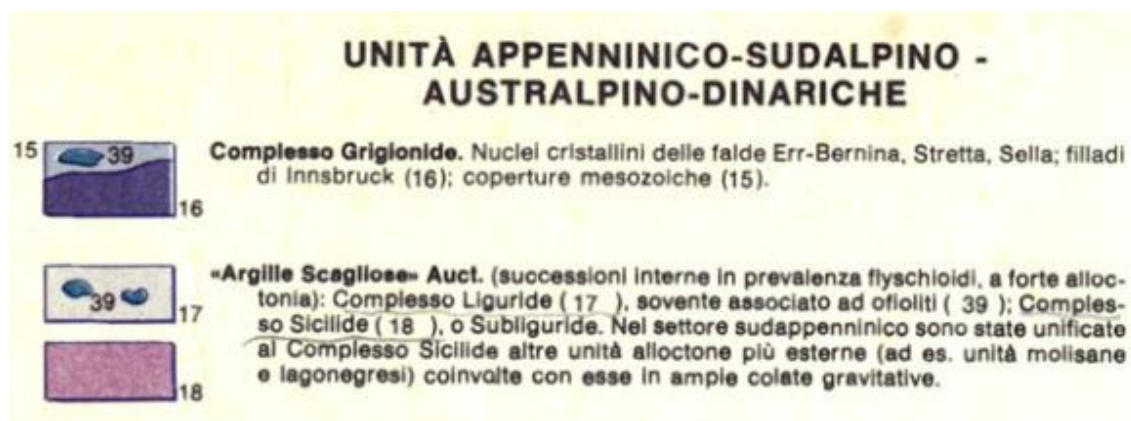
Figura 3: Carta Tettonica d’Italia – Progetto finalizzato GEODINAMICA CNR – sca 1:500.000
