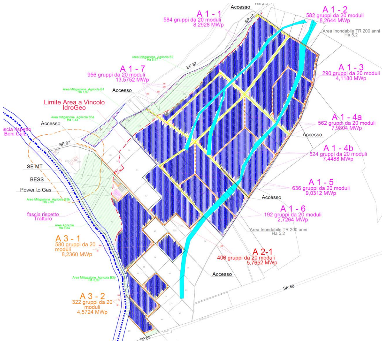
Fig 3.16 – Layout generale della piattaforma
