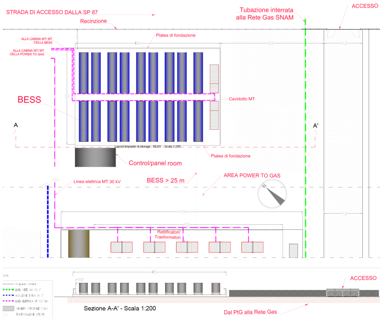
Fig. 3.23 – Layout BESS
