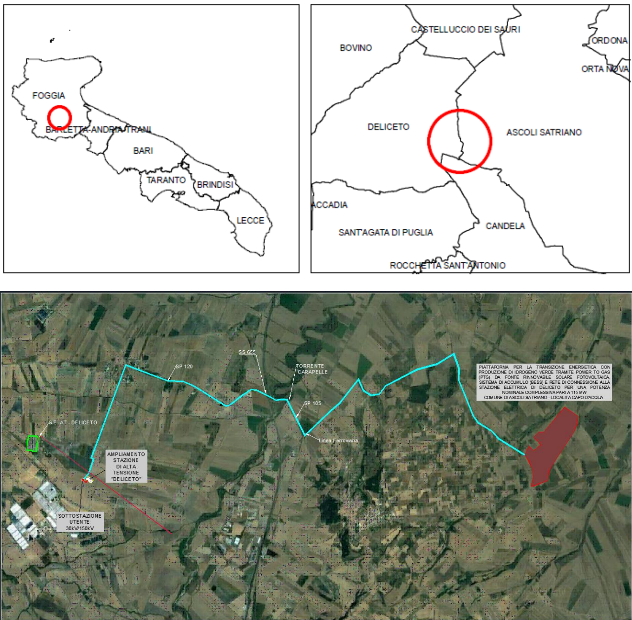
Fig. 2.3 - Inquadramento Territoriale della Piattaforma e della Rete di connessione alla Stazione Elettrica di Deliceto
