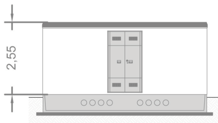
Prospetto longitudinale
